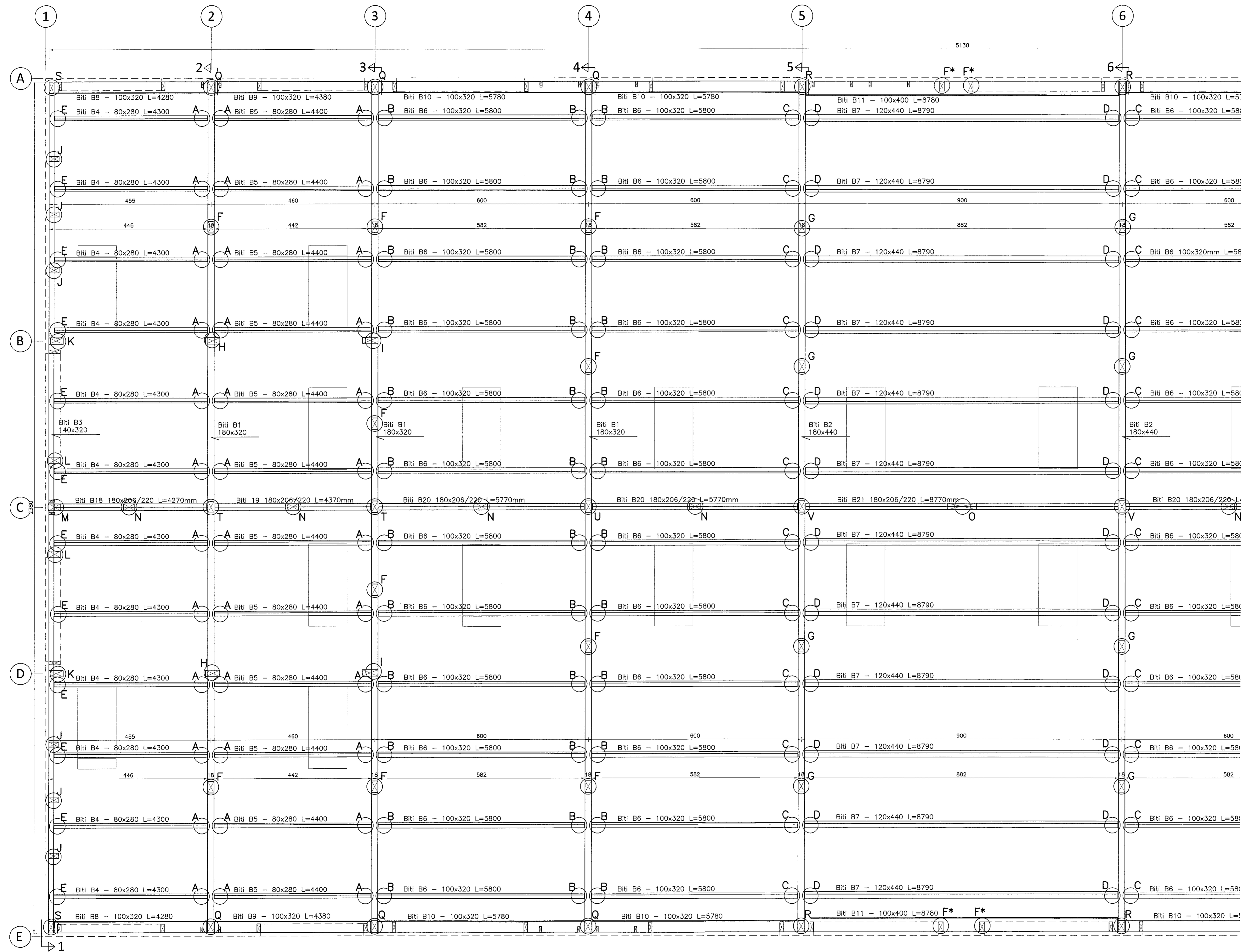
Grunnmynd þakviða (milli lína 1-6) 1:50
