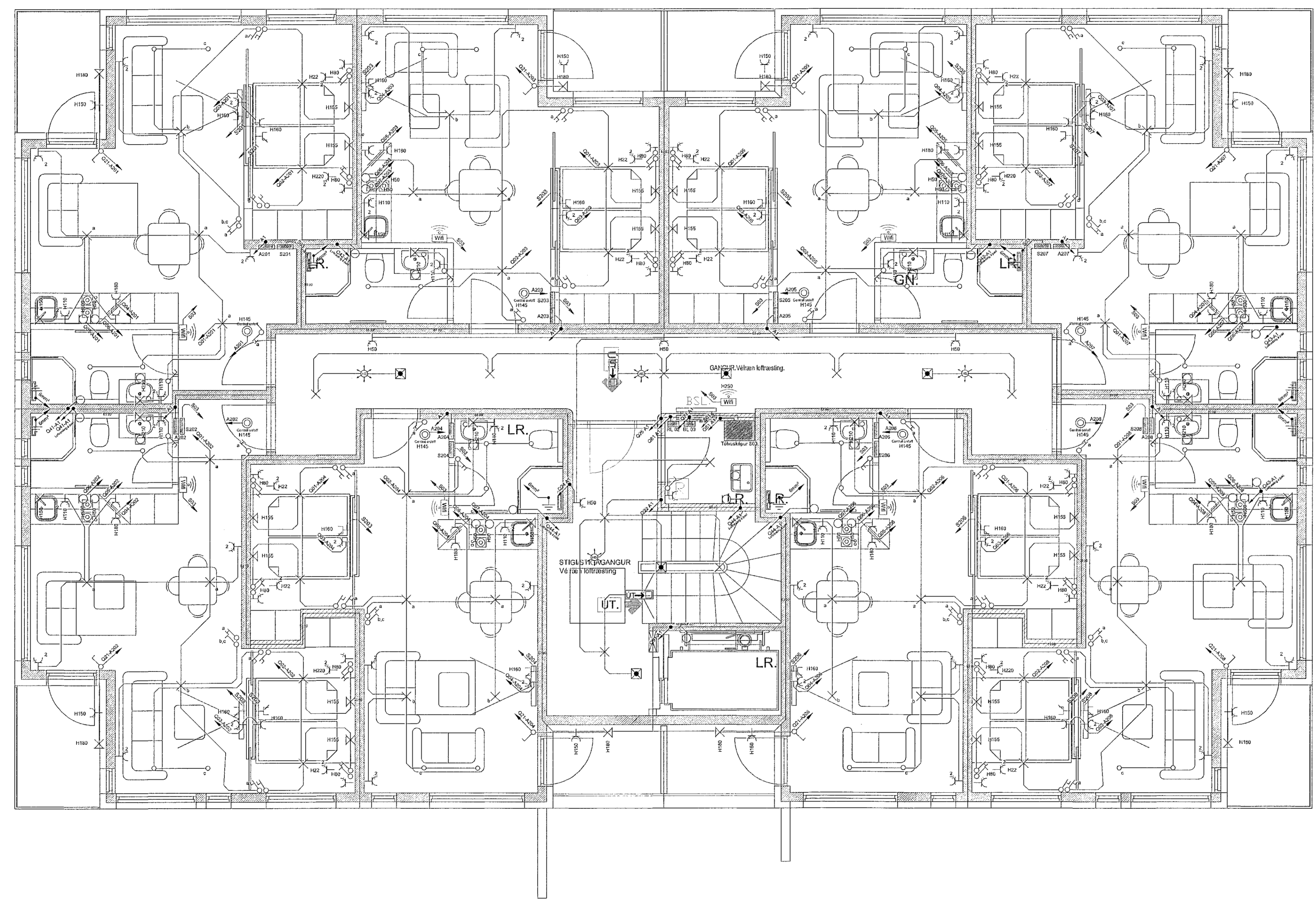
GRUNNMYND 2 HÆÐ
