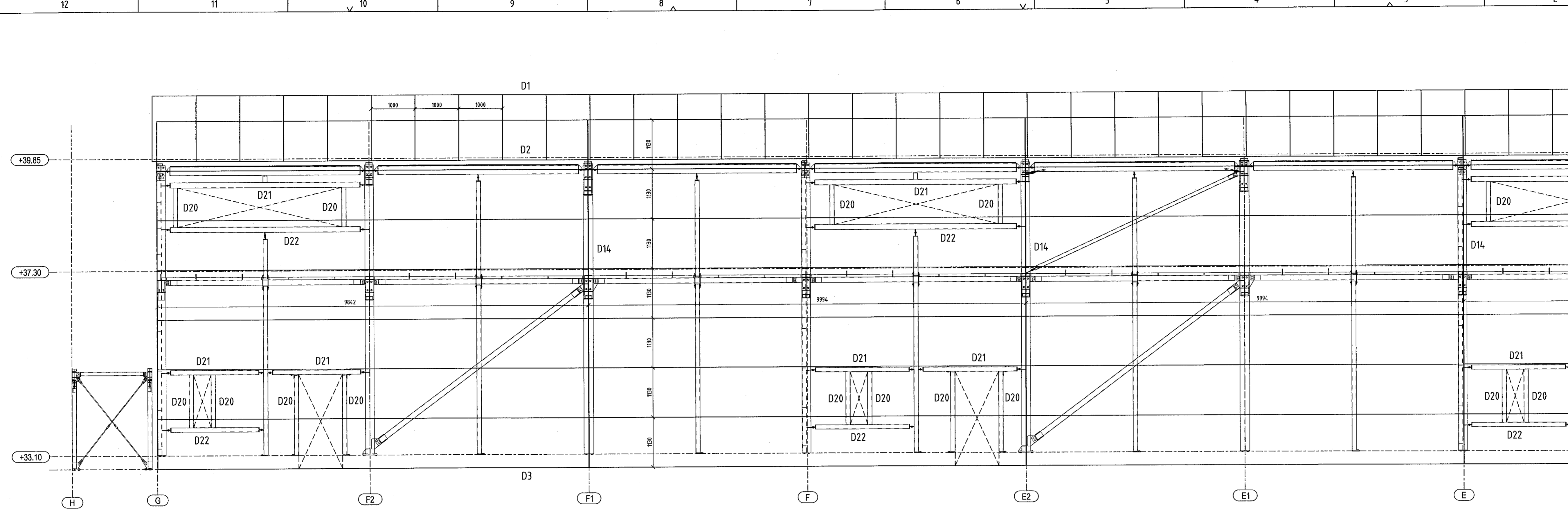
LANGHLIÐ LÍNA 1 - ÚTLIT NORÐURHLIÐ 1:50
