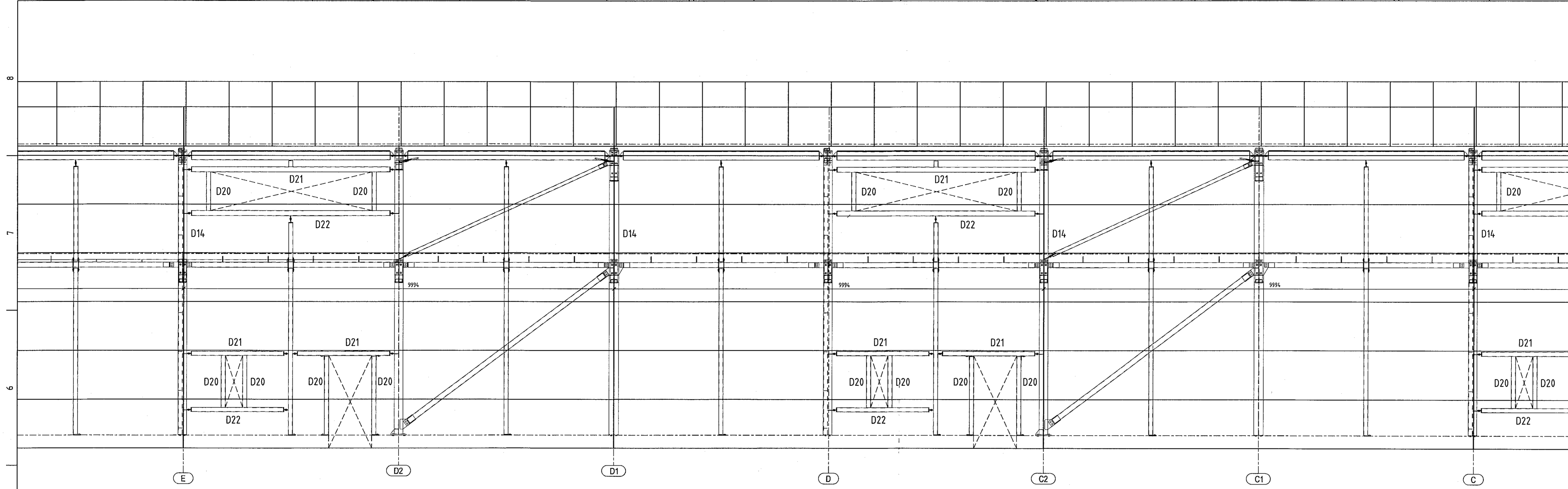
LANGHLID LÍNA 1 - ÚTLIT NORÐURHLID 1:50
