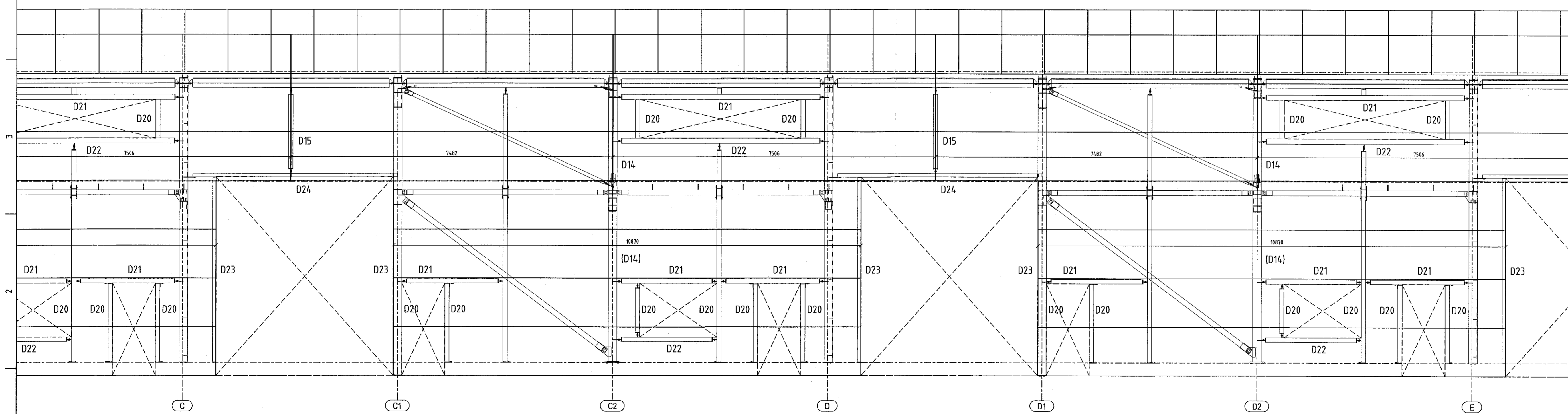
LANGHLID LÍNA 4 - ÚTLIT SUÐURHLID 1:50
