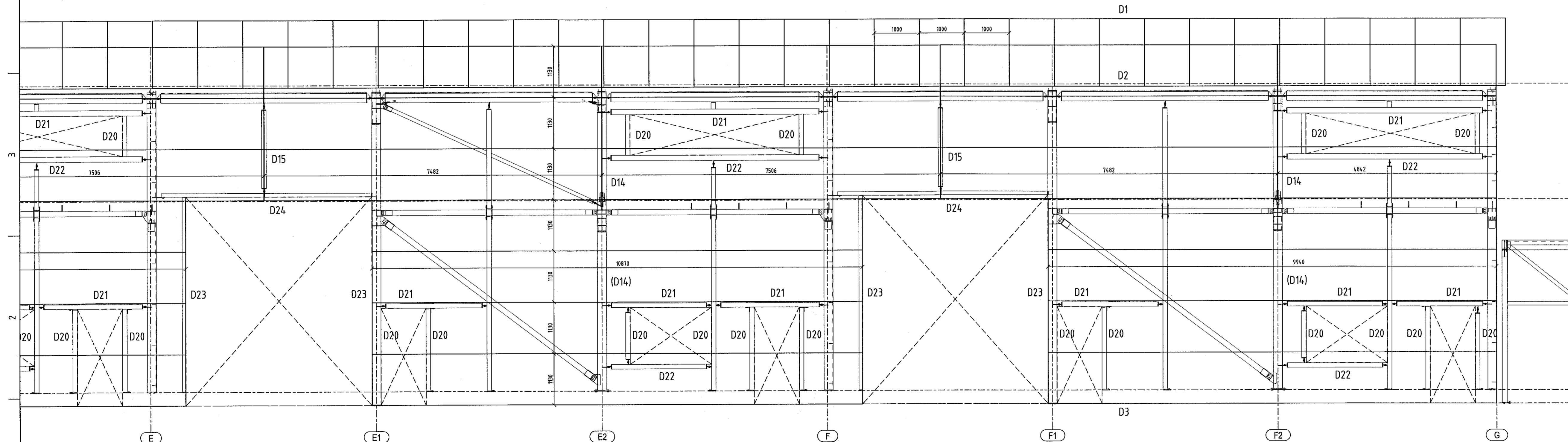
LANGHLIÐ LÍNA 4 - ÚTLIT SUÐURHLIÐ 1:50
