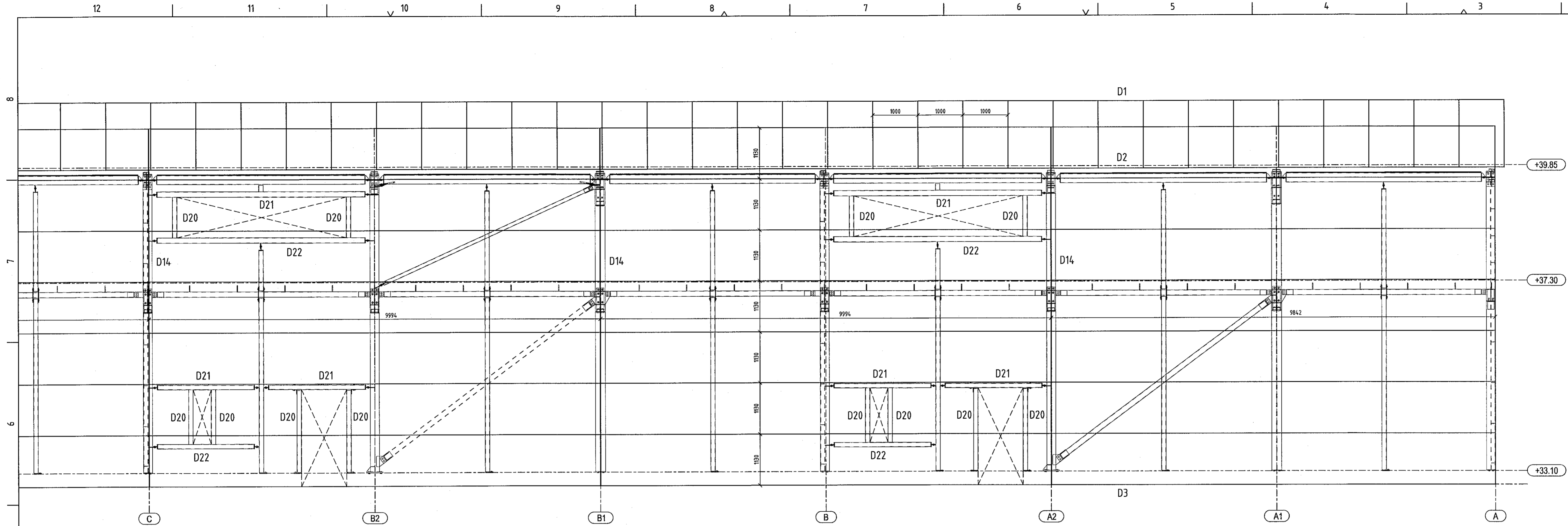
LANGHLIÐ LÍNA 1 - ÚTLIT NORÐURHLIÐ 1:50
