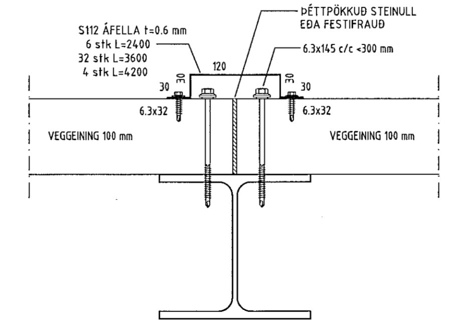
SAMSEYTI VEGGEININGA - D14
