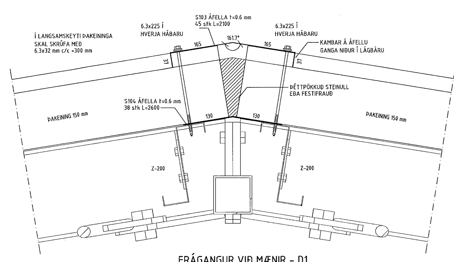
FRÁGANGUR VID MÆNIR - D1
