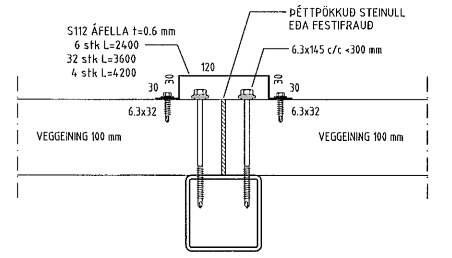
SAMSEYTI VEGGEININGA - D15
