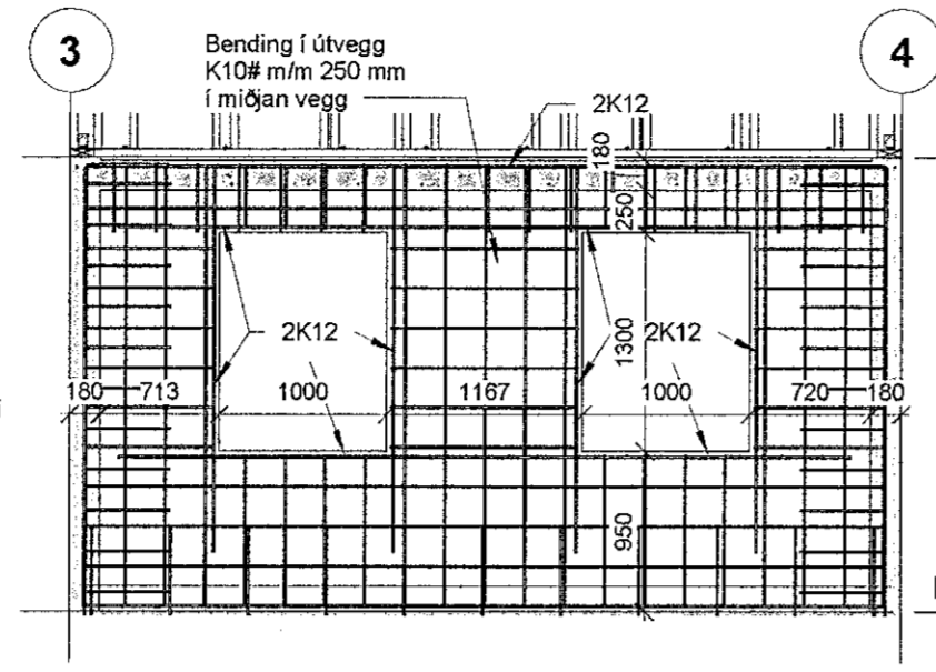
2 Burðarveggur 02 1 : 50
