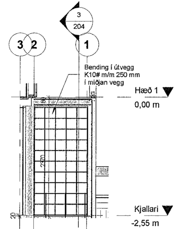
5 Burðarveggur 05 1 : 50
