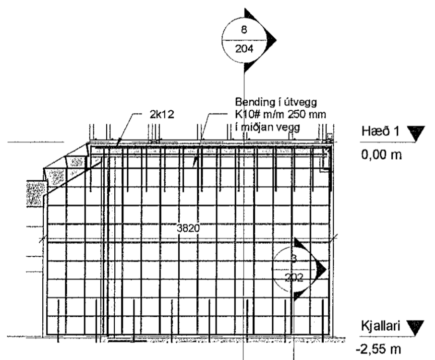
4 Burðarveggur 04 1 : 50
