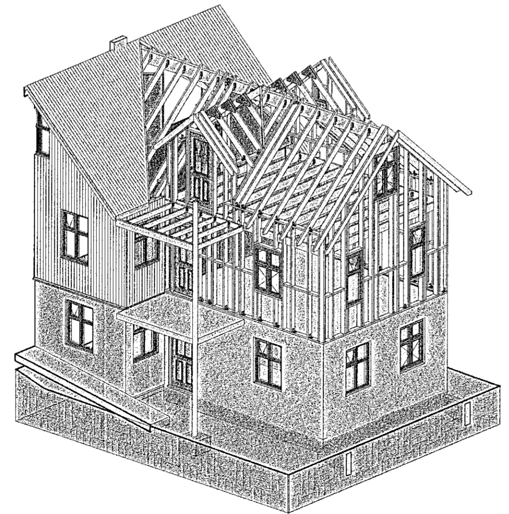
3D burðarvirki - Ásýnd
