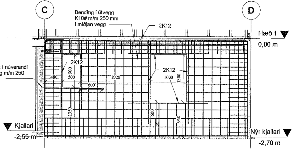
1 Burðarveggur 01 1 : 50
