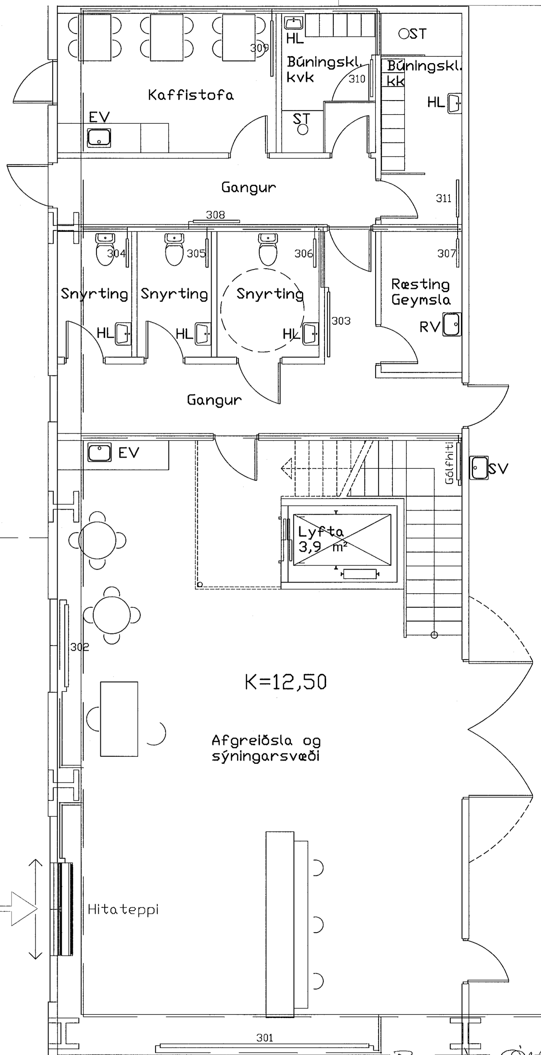
Grunnmynd 1:50
