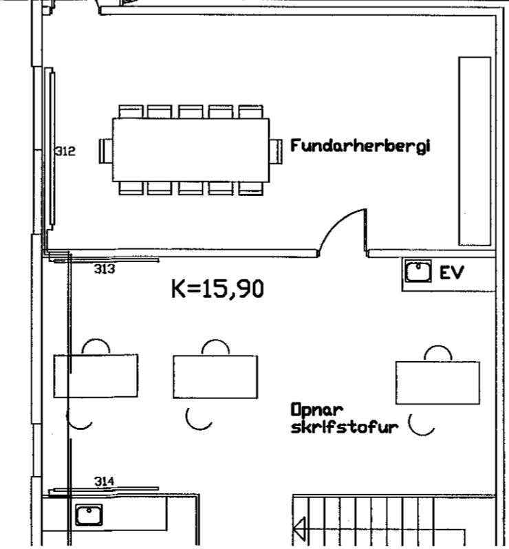
Grunnmynd 1:100, 2 hæð
