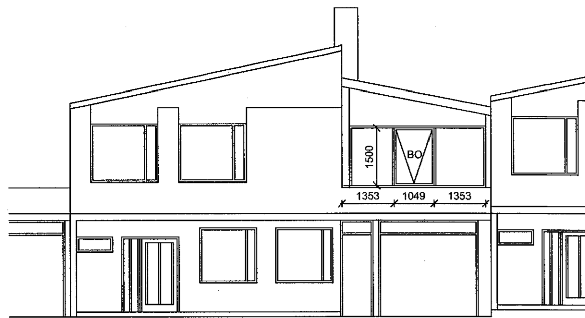
5 ÁSÝND - Norðurhlíð - 1:100
