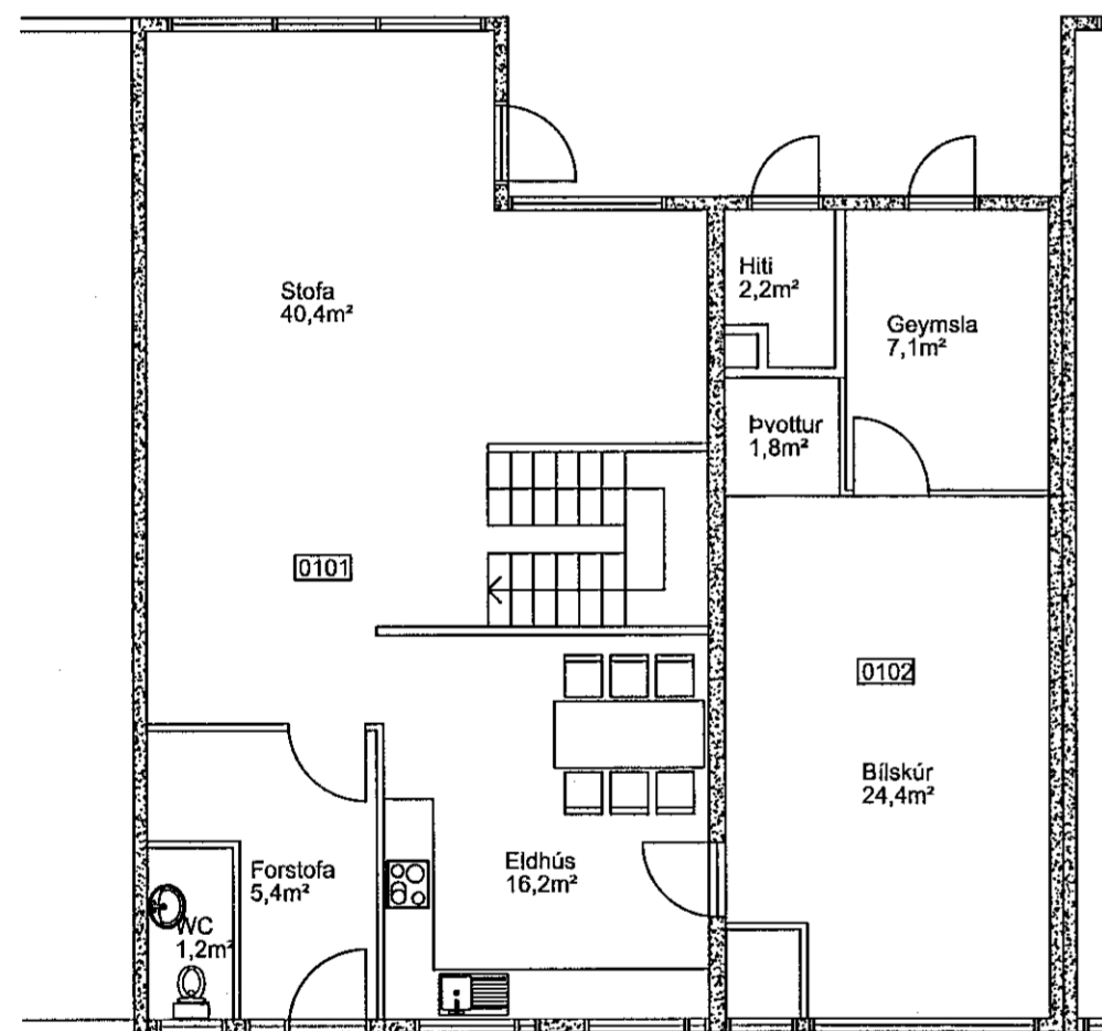
7 GRUNNMYND - 1. hæð - 1:100
