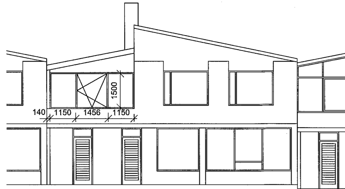
6 ÁSÝND - Suðurhlíð - 1:100
