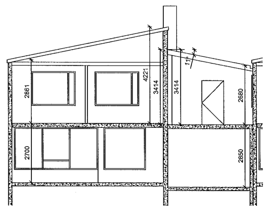
9 SNID - 1:100
