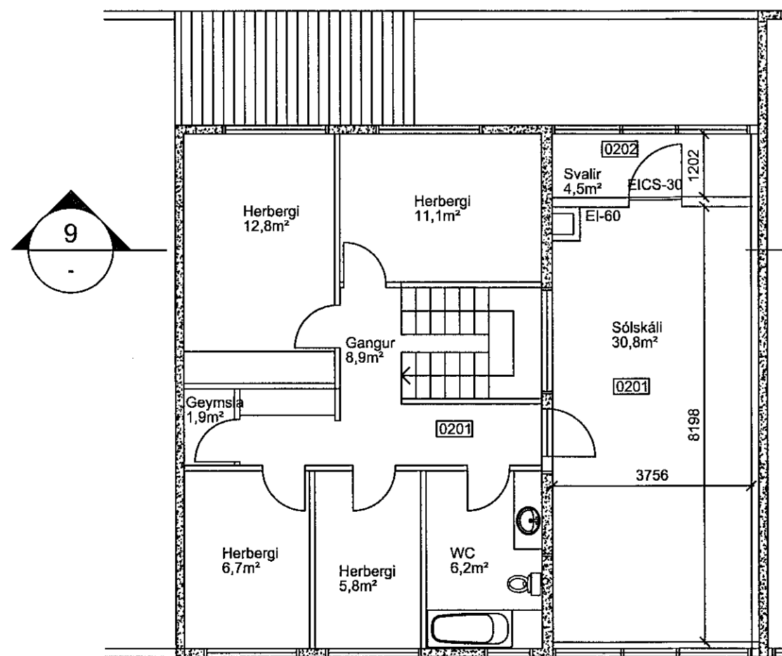
8 GRUNNMYND - 2. hæð - 1:100
