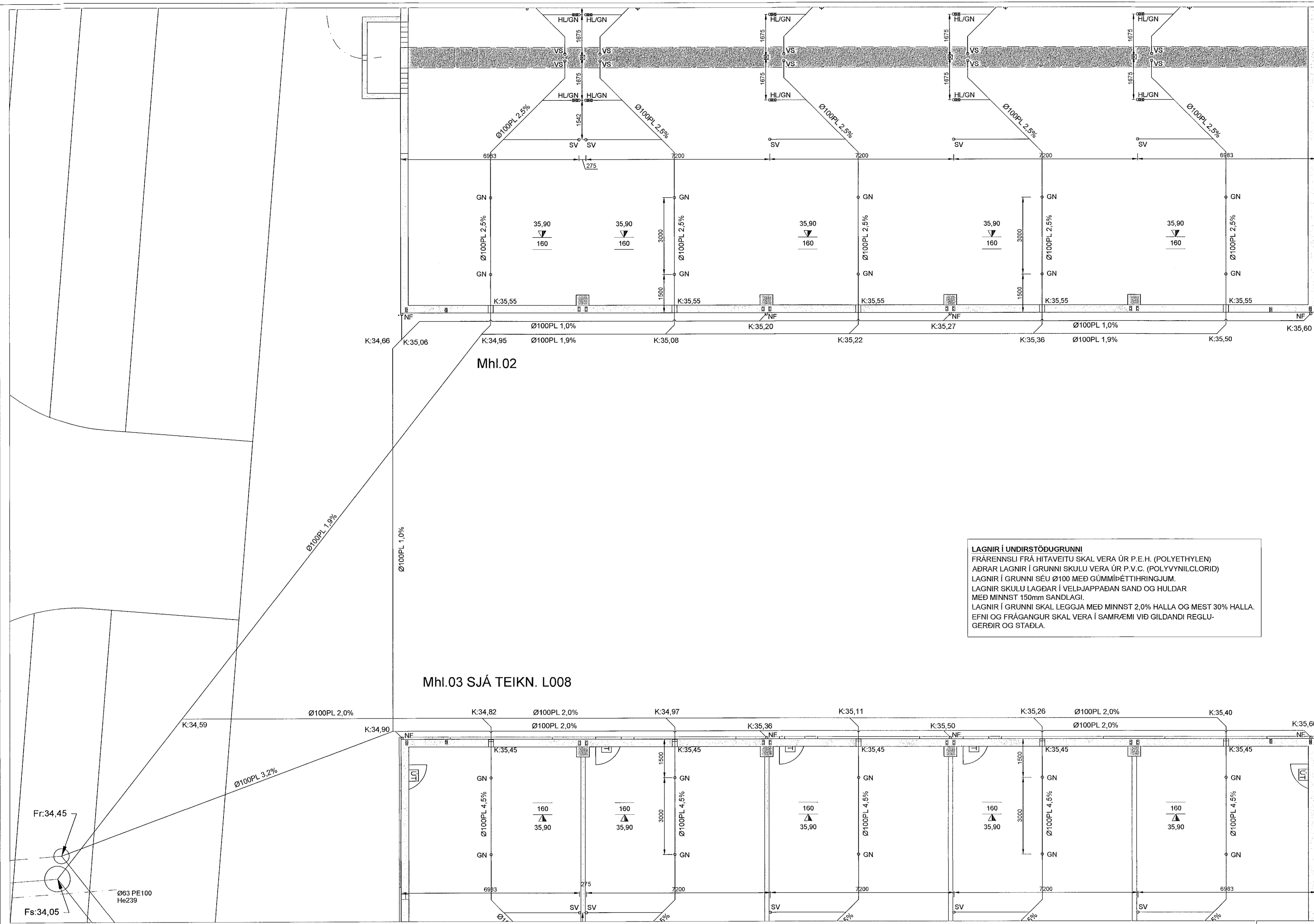
GRUNNMYND - FRÁRENNSLI 1:75 (A1)
