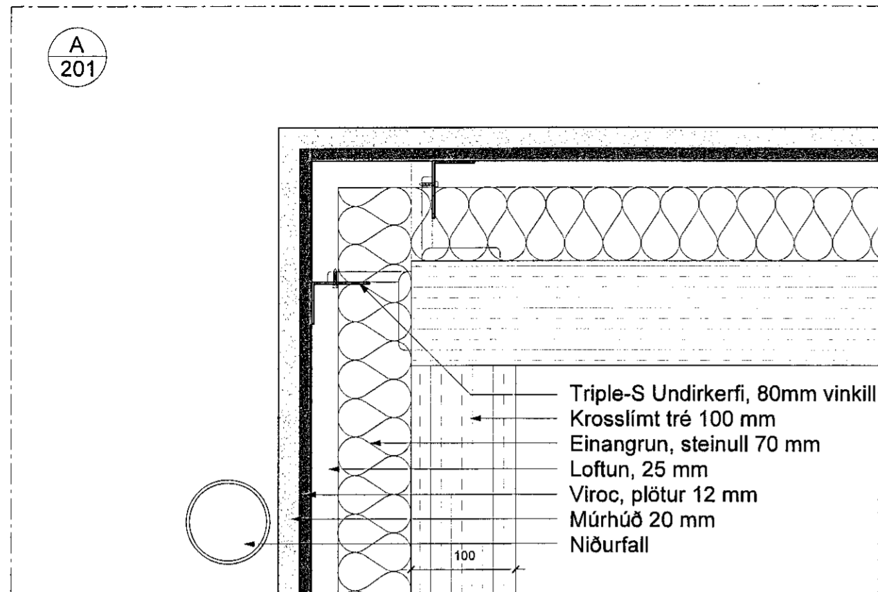
Lárétt deili A 1:5
