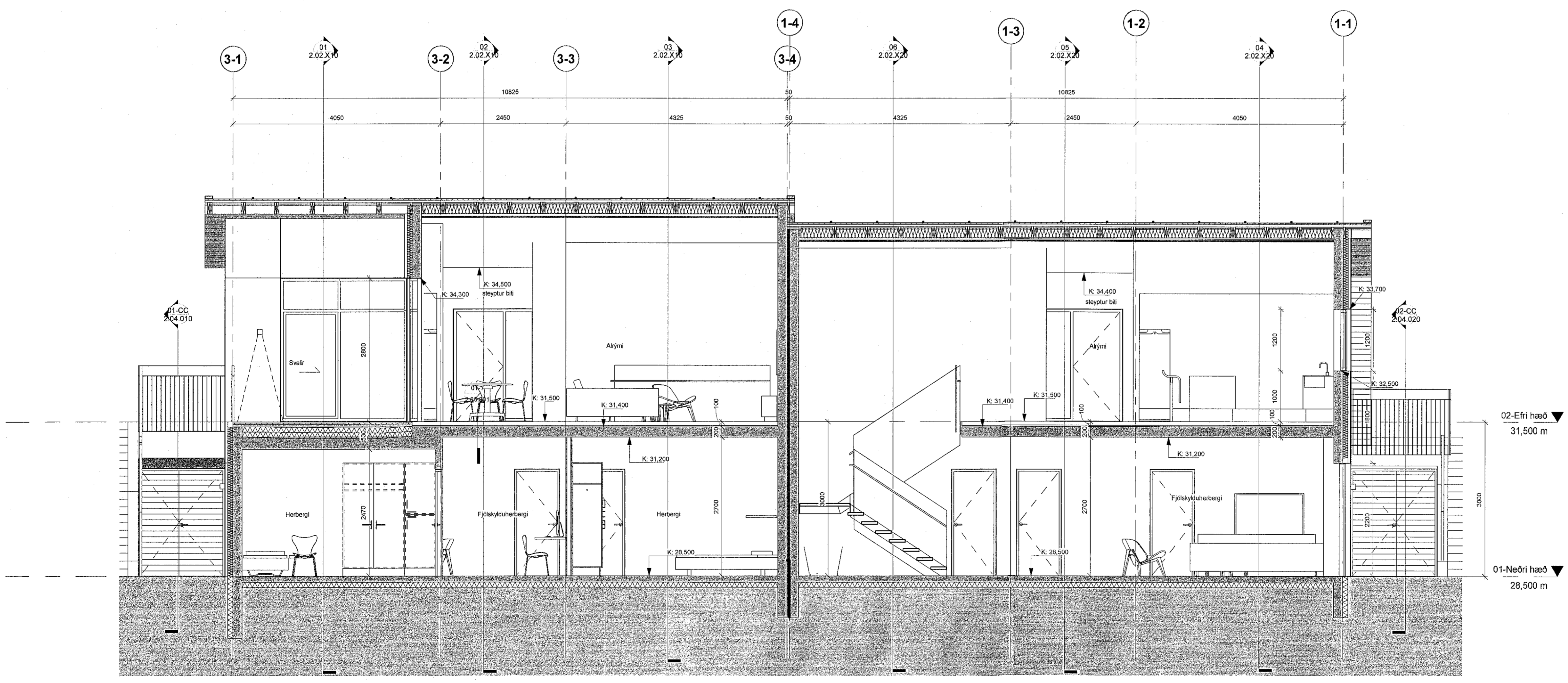
08 Snið 08 1:50
