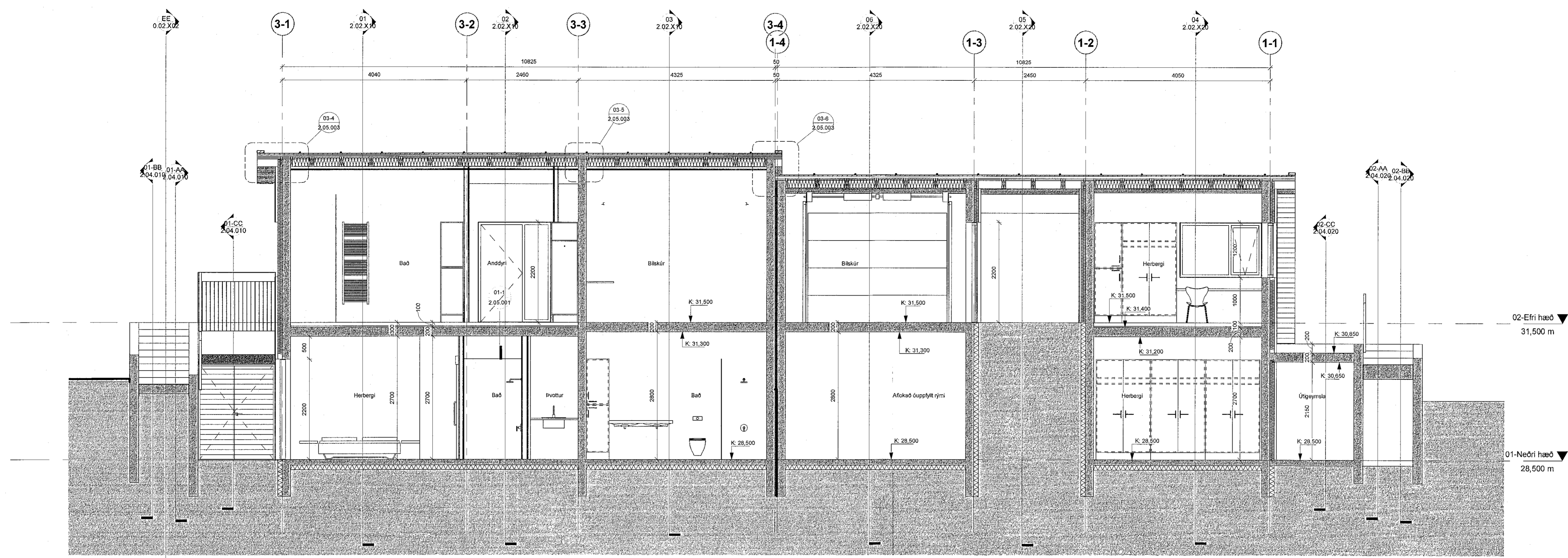
07 Snið 07 1:50
