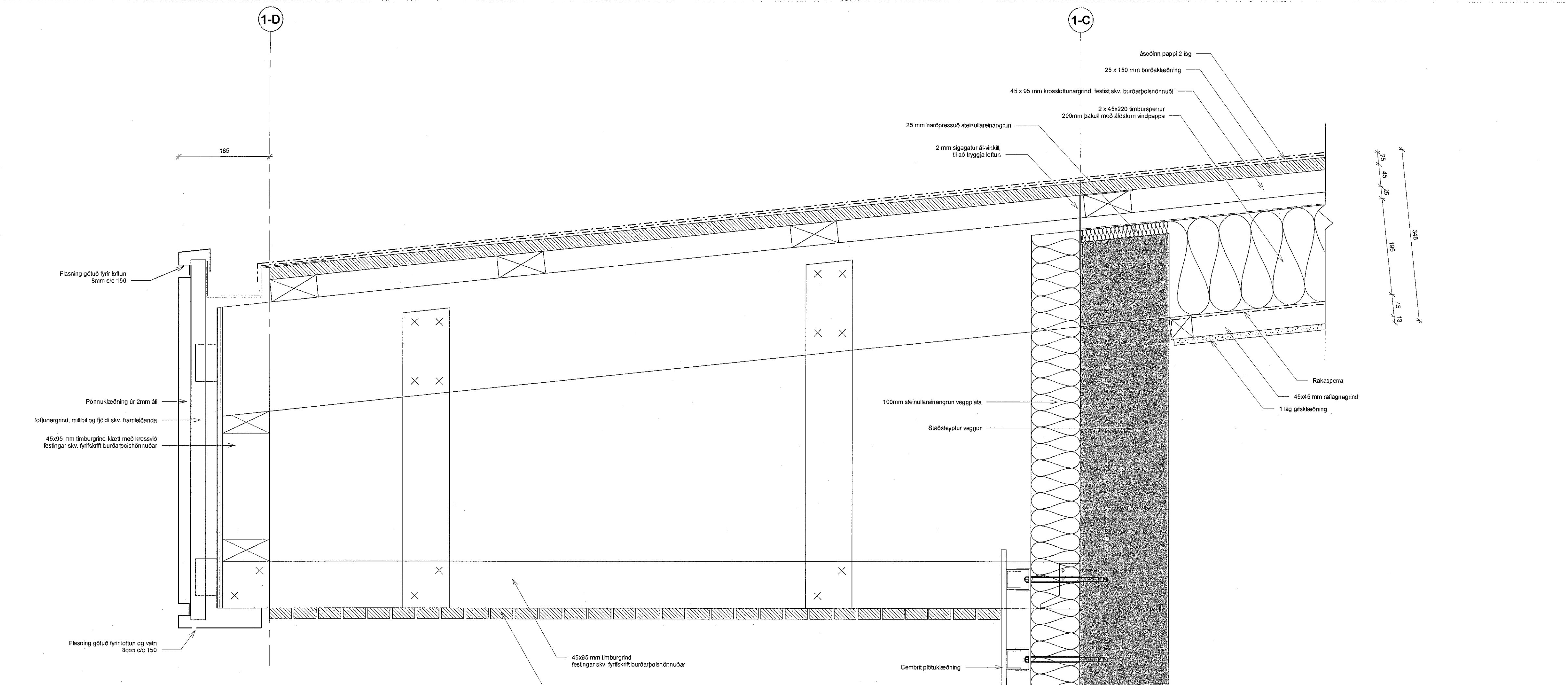
04-1 Deili 04-1 - Lóðrétt deili þak inngangur 1:5
