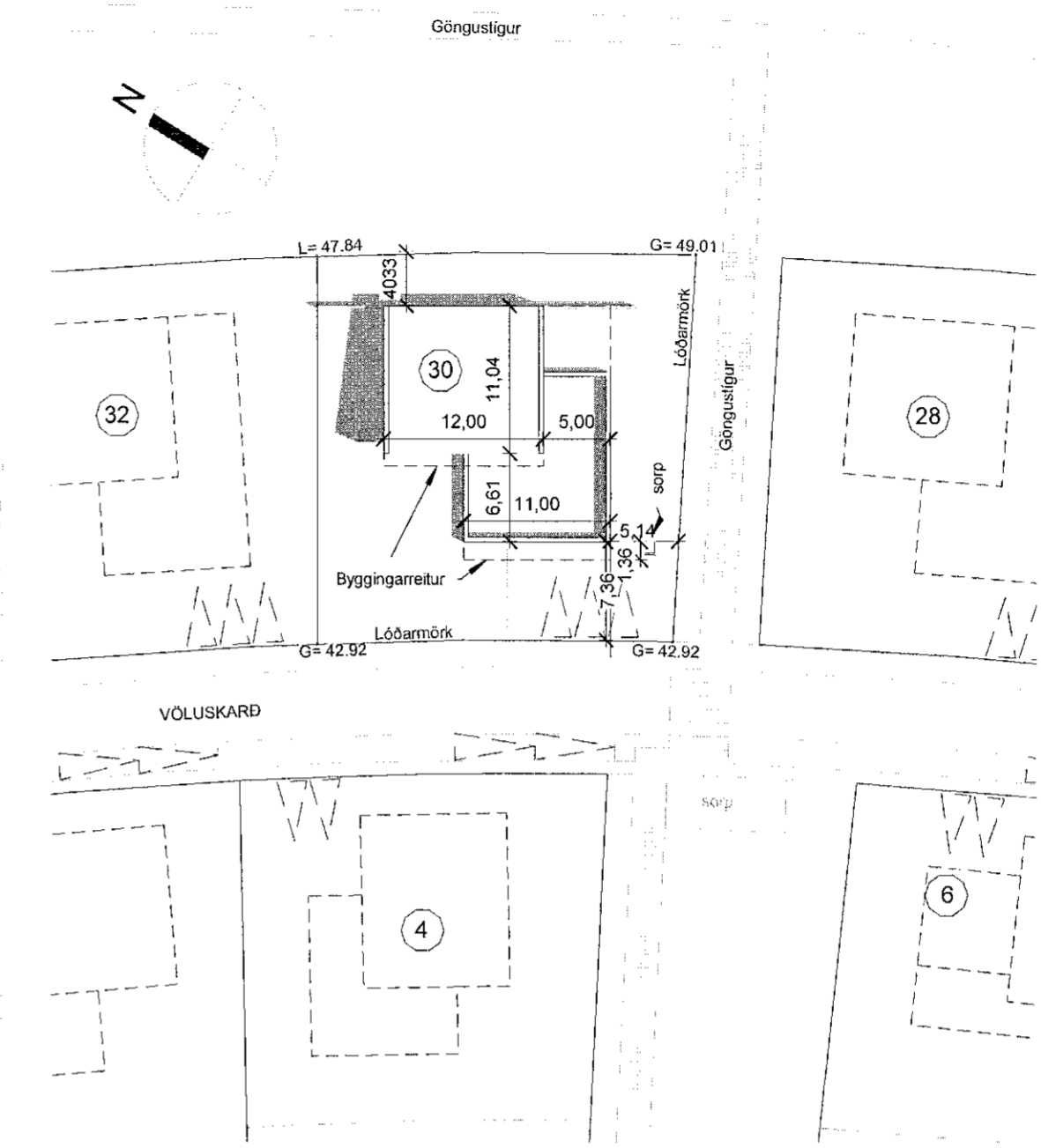
Afstöðumynd 1 : 500
