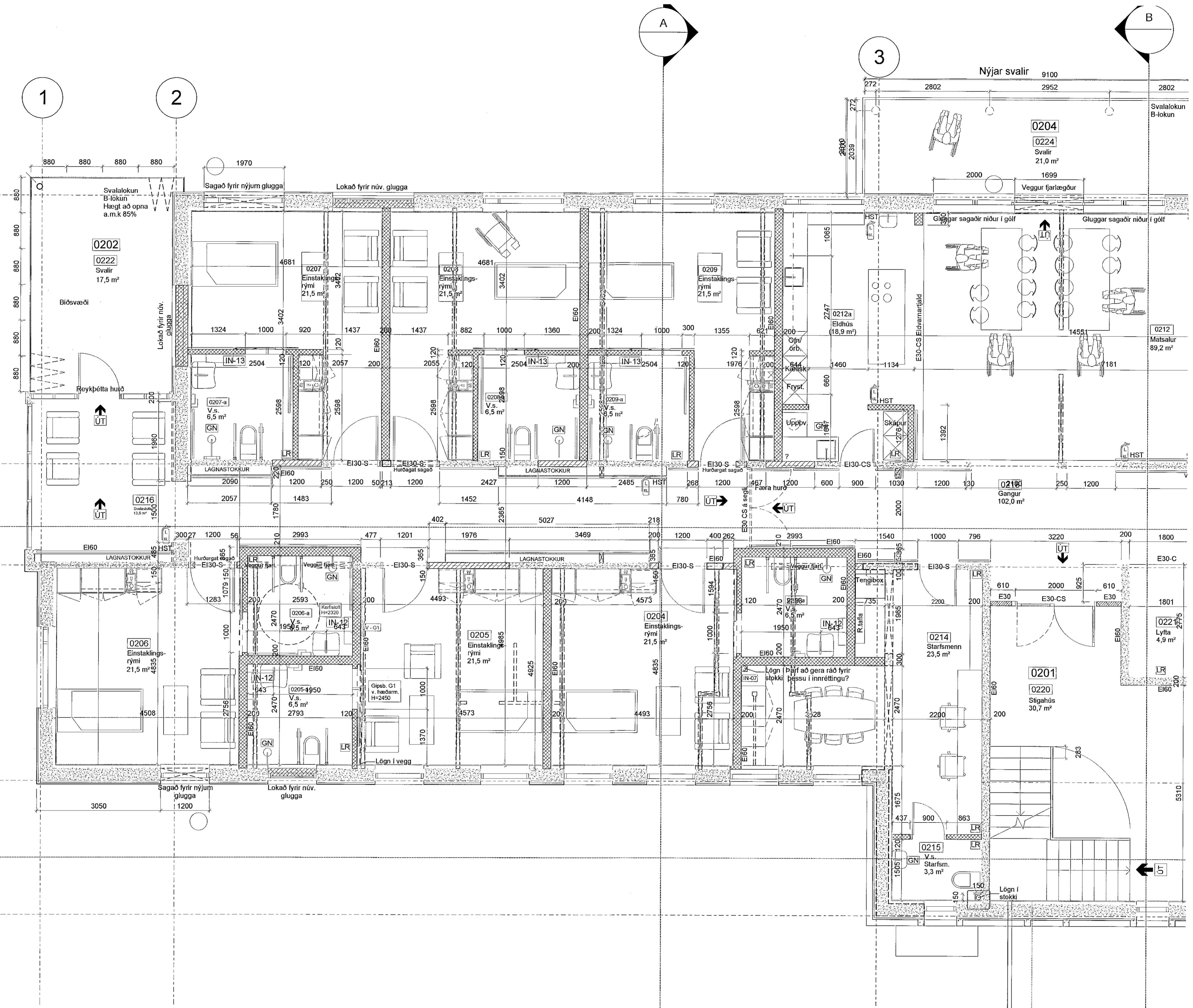
GRUNNMYND 2. HÆÐAR 1:50
