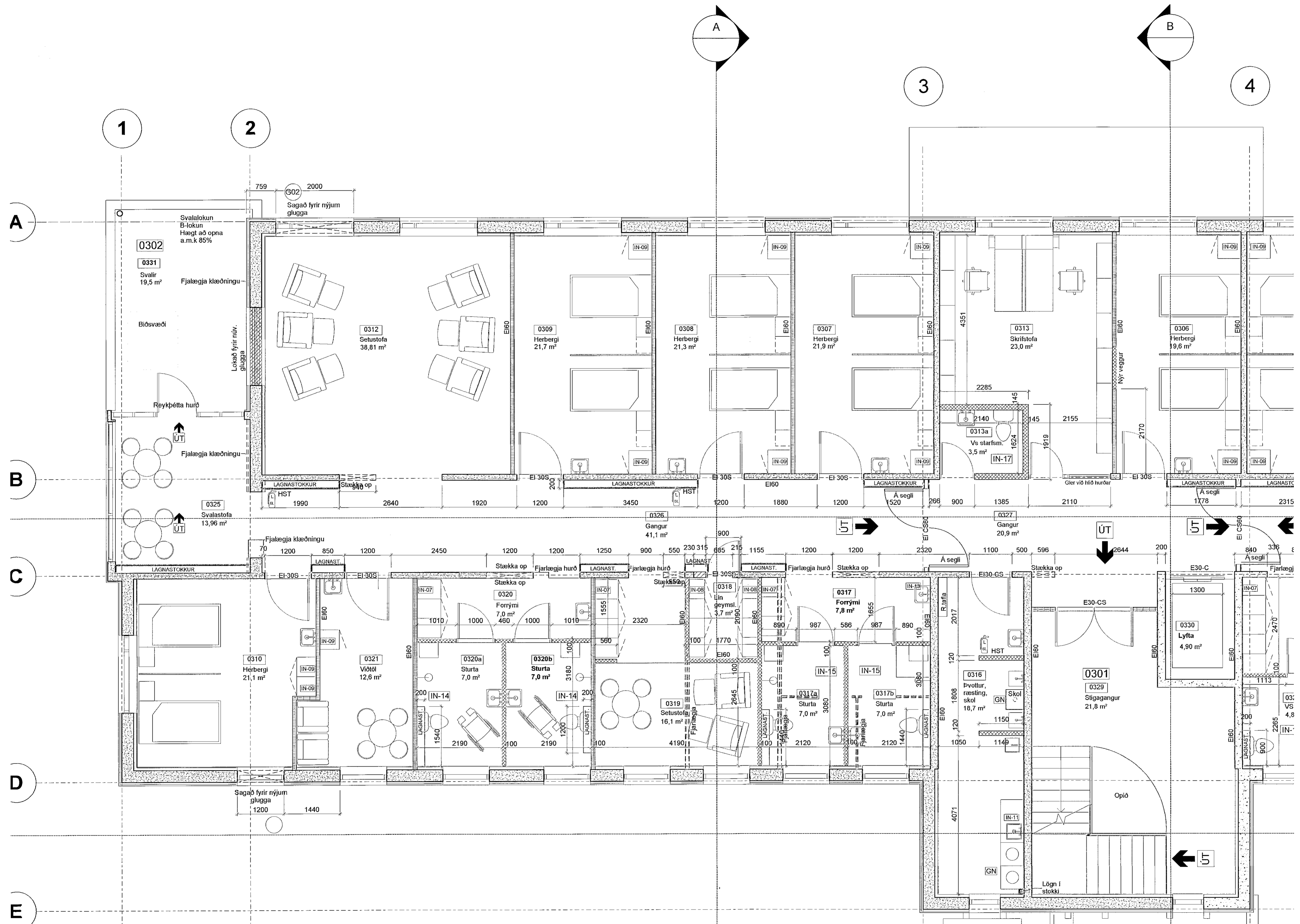
GRUNNMYND 3. HÆÐAR 1:50
