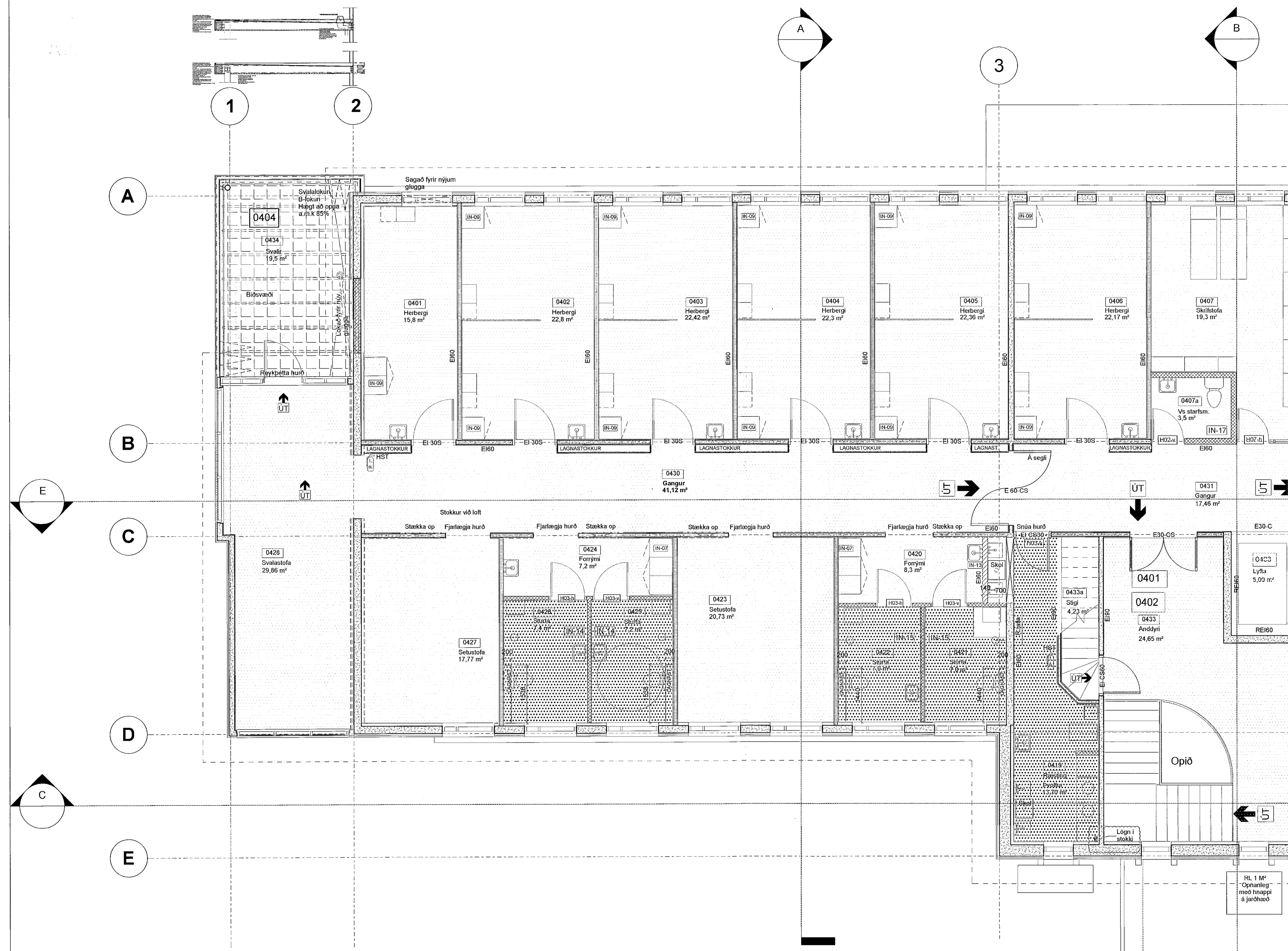
GRUNNMYND 4. HÆÐAR (1 af 2) 1:50
