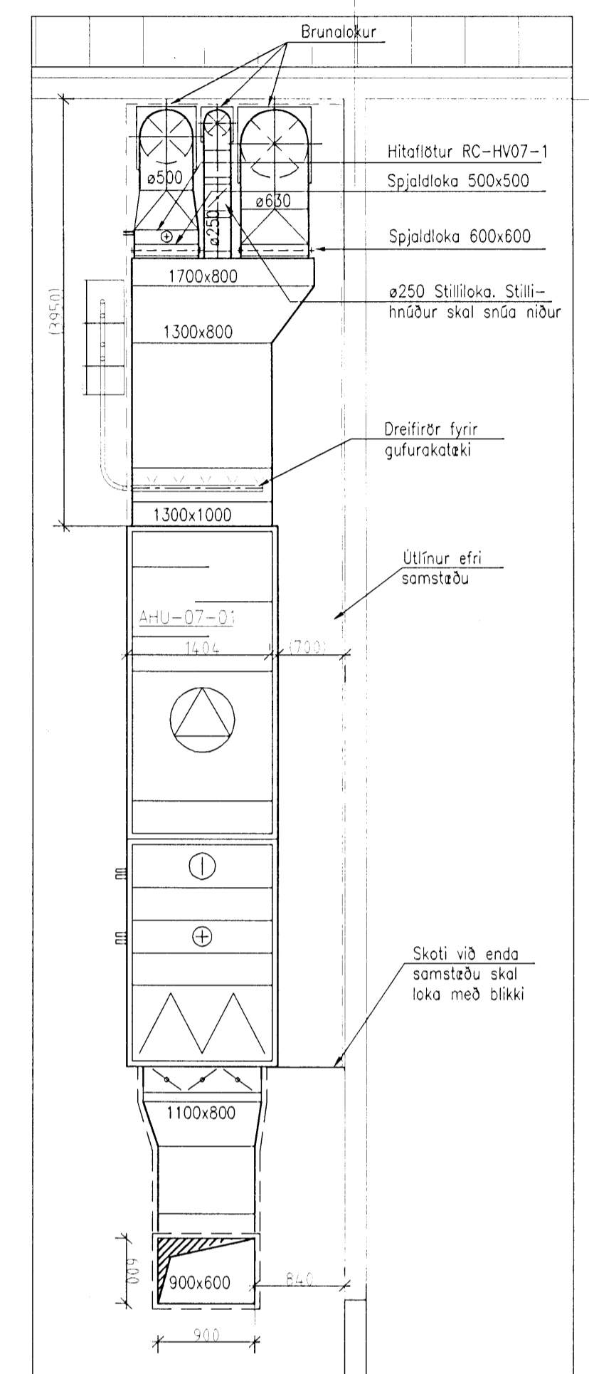
Grunnmynd - Samstæða AHU-07-01 Mkv. 1:50
