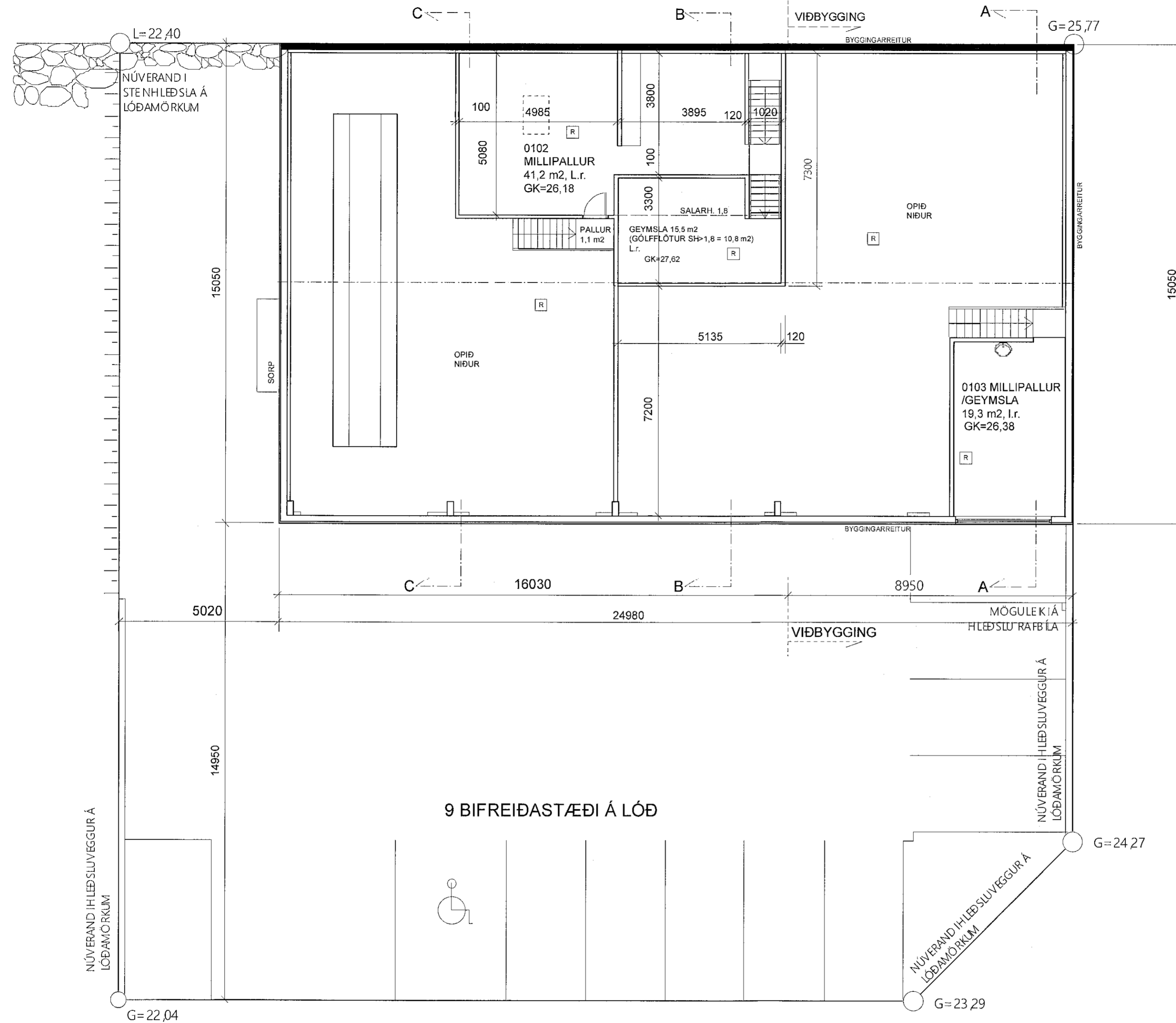
Grunnmynd 2. hæð
