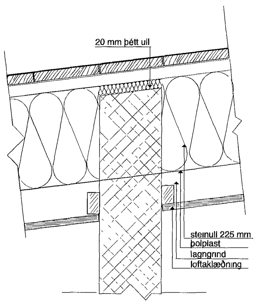
D-7 lóðrétt snið í þak
