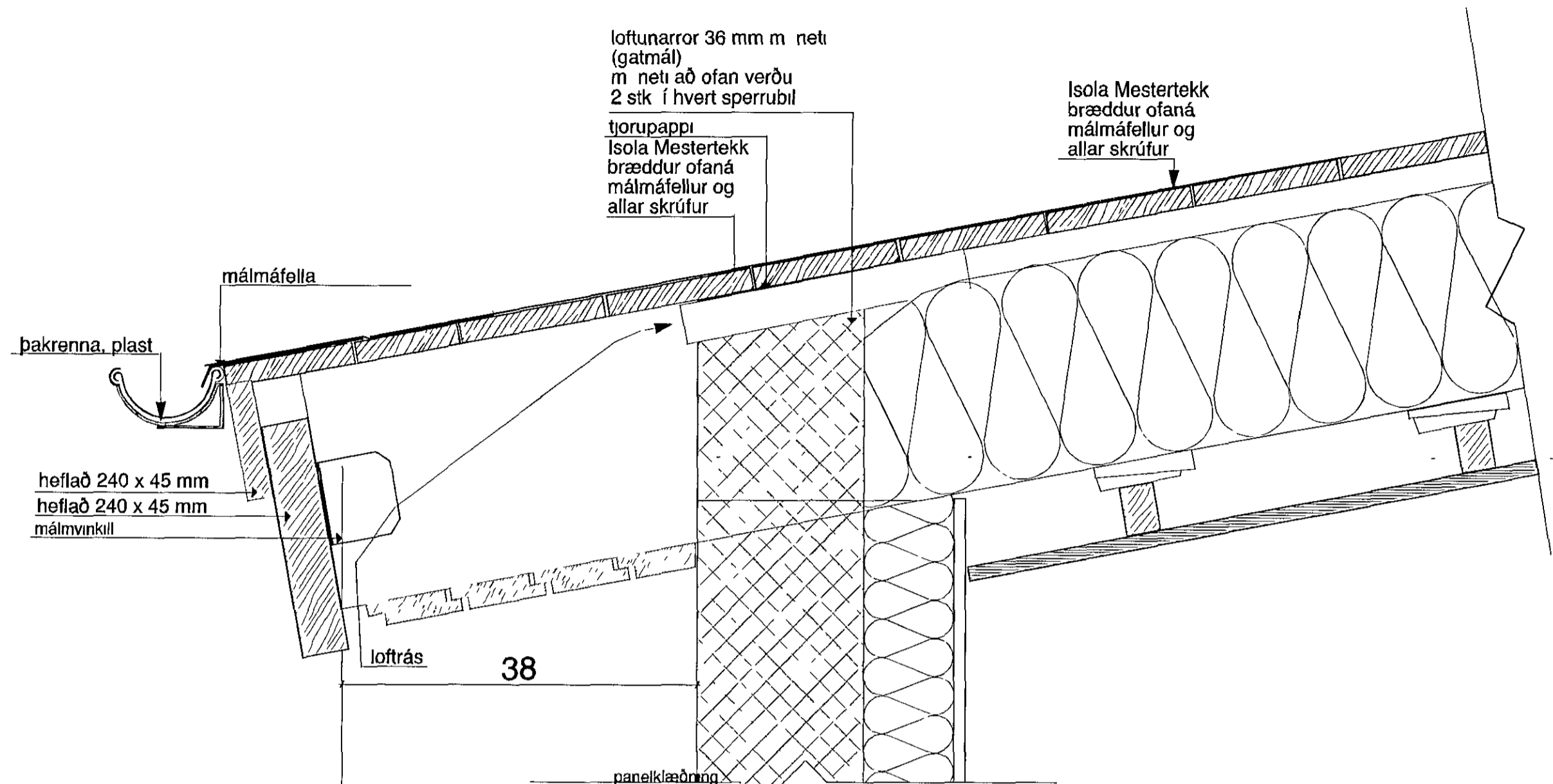
D-2 lóðrétt snið í þakkant
