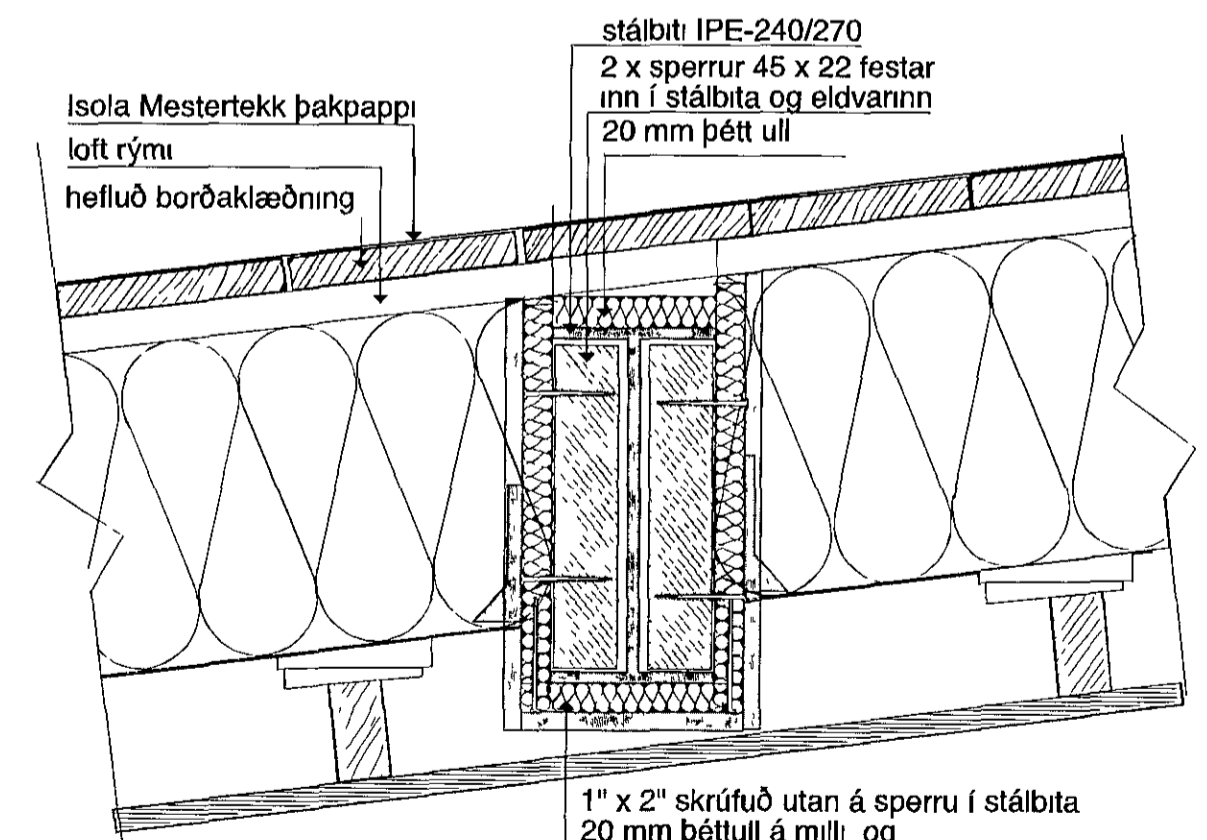
D-4 lóðrétt snið í þak/stálbita
