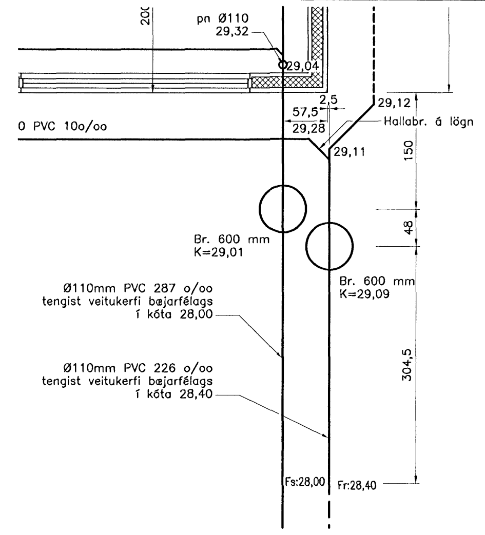
Tenging við veitukerfi 1:50
