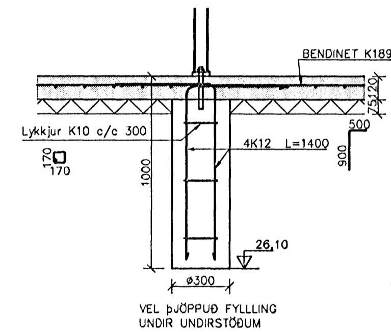
DEILI E 1:20
