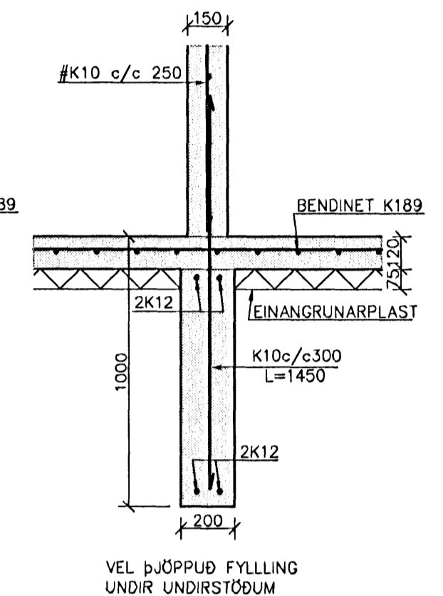
DEILI C 1:20
