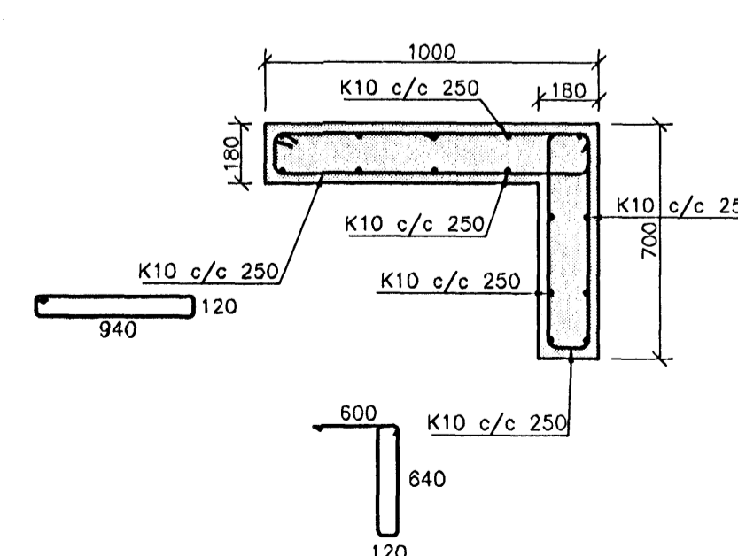
DEILI H 1:20
