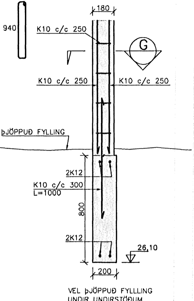
DEILI D 1:20
