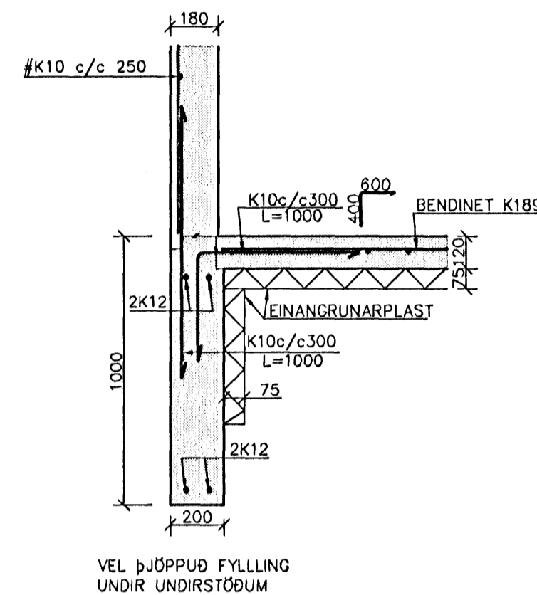
DEILI E 1:20
