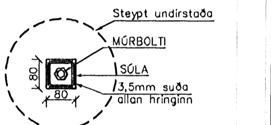
DEILI F 1:10
