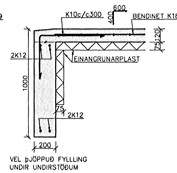
DEILI B 1:20
