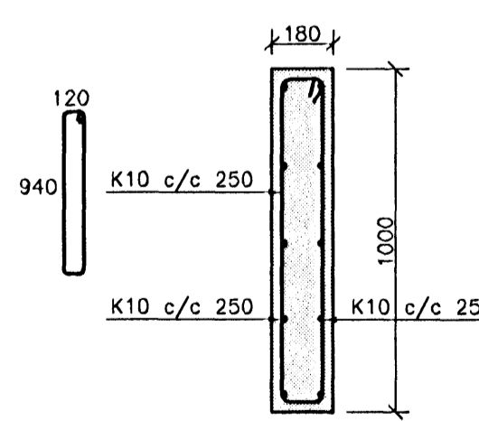
DEILI G 1:20
