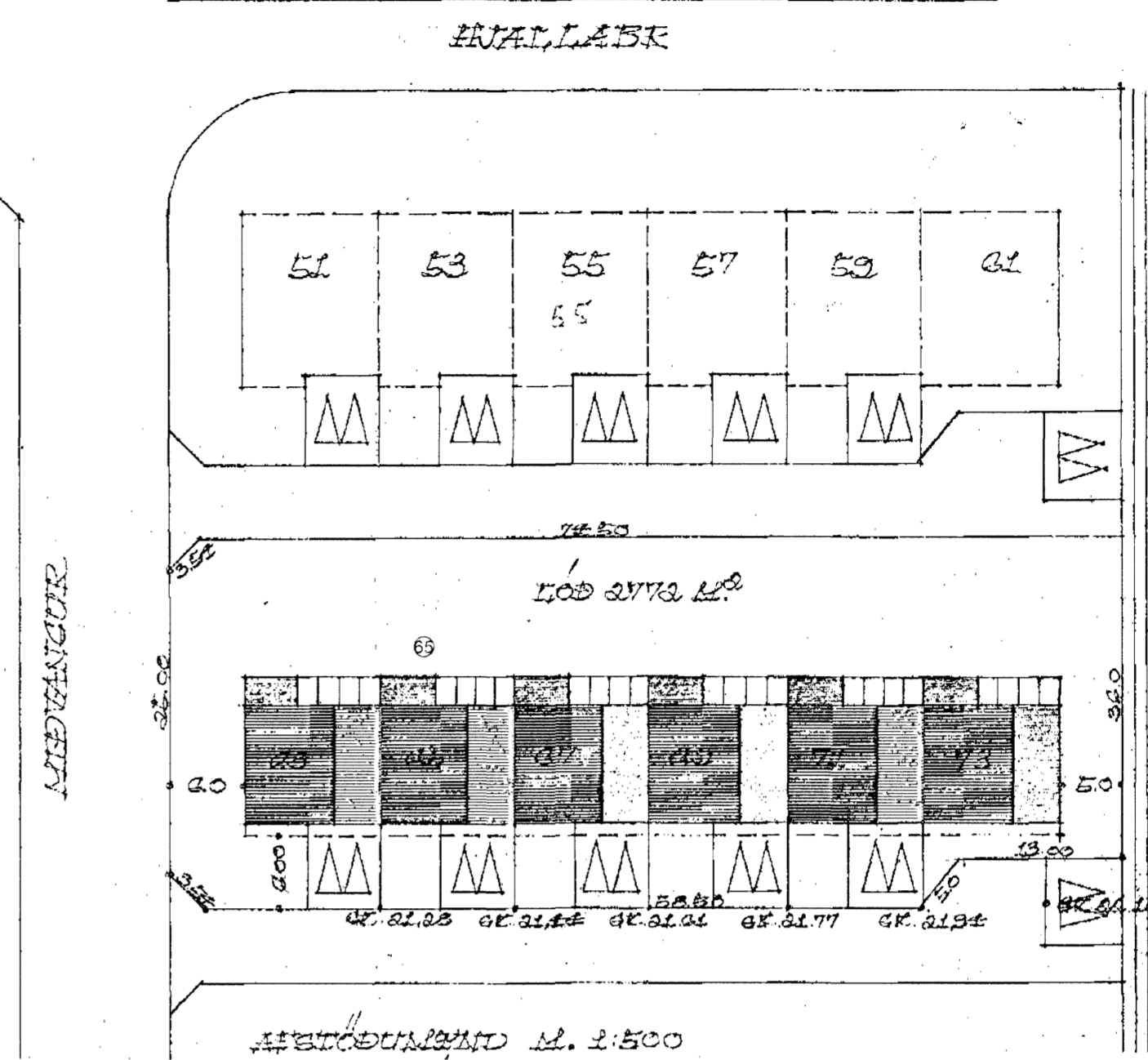
AFSTÖÐUMYND 1:500
