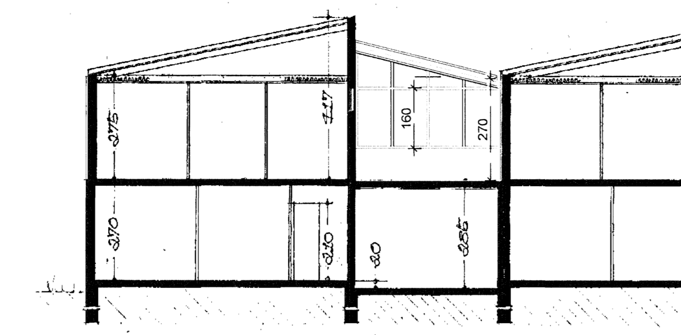
SKURÐUR A-A
