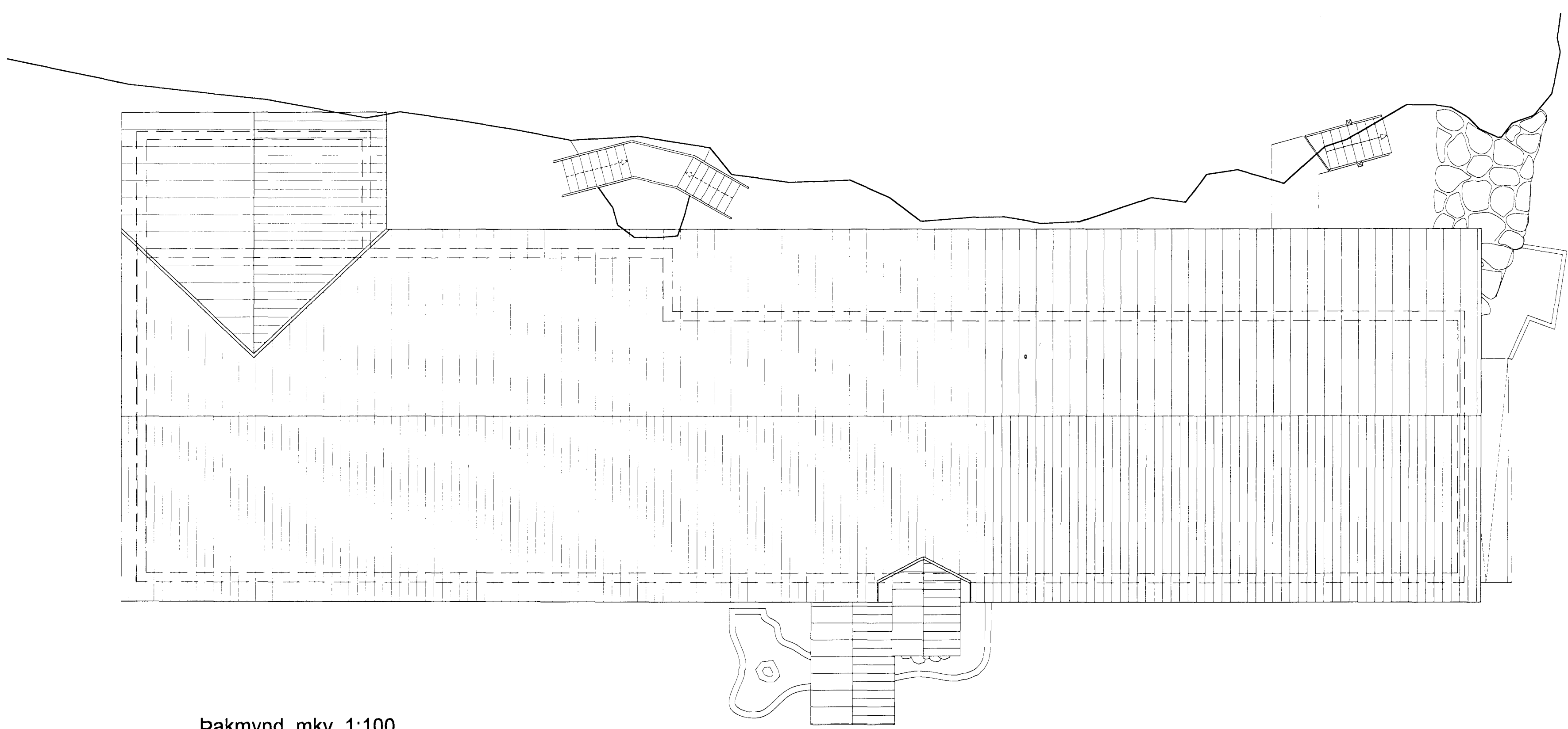
Þakmynd mkv. 1:100.
