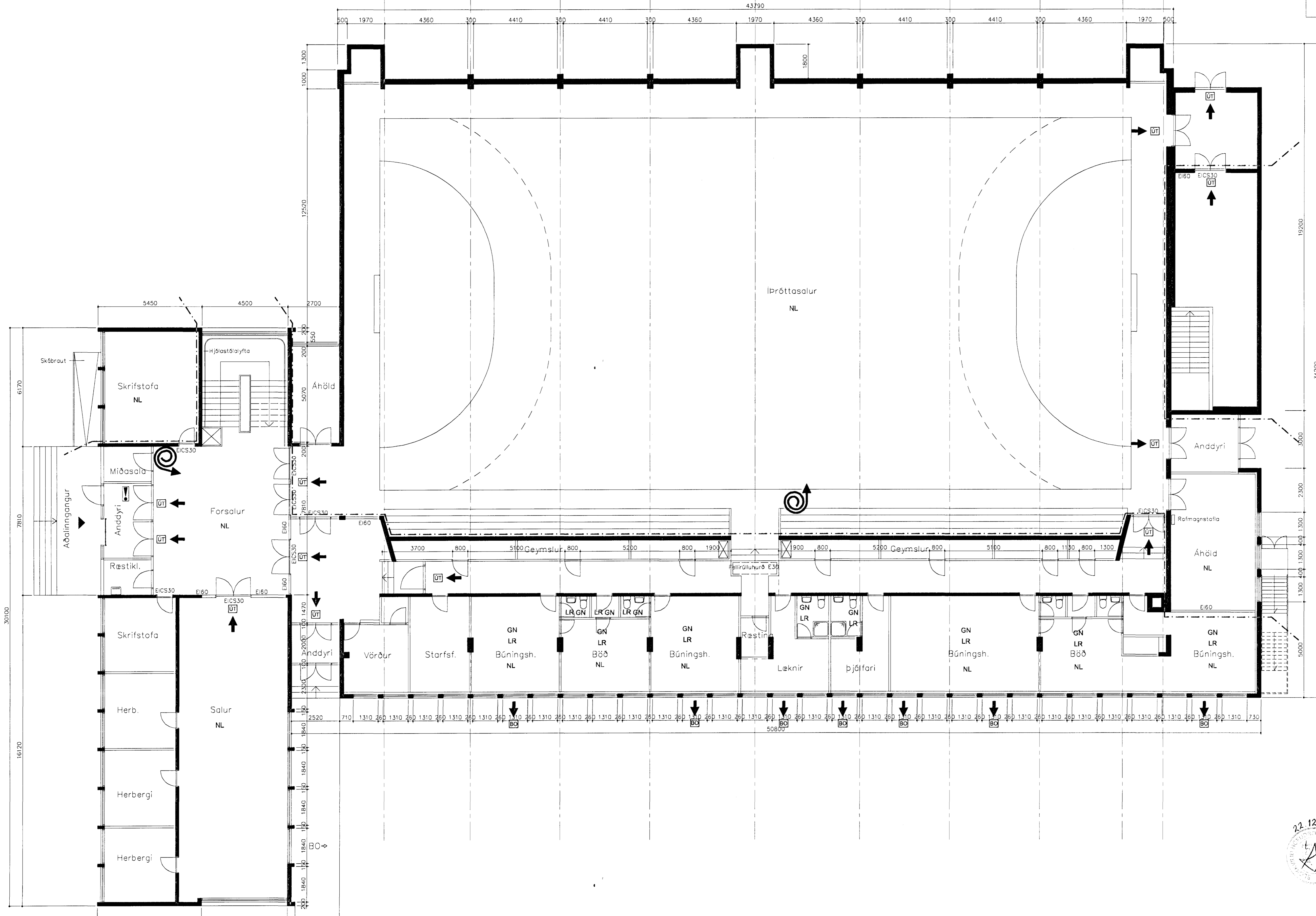
GRUNNMYND, 1.HÆÐ, MKV. 1:100
