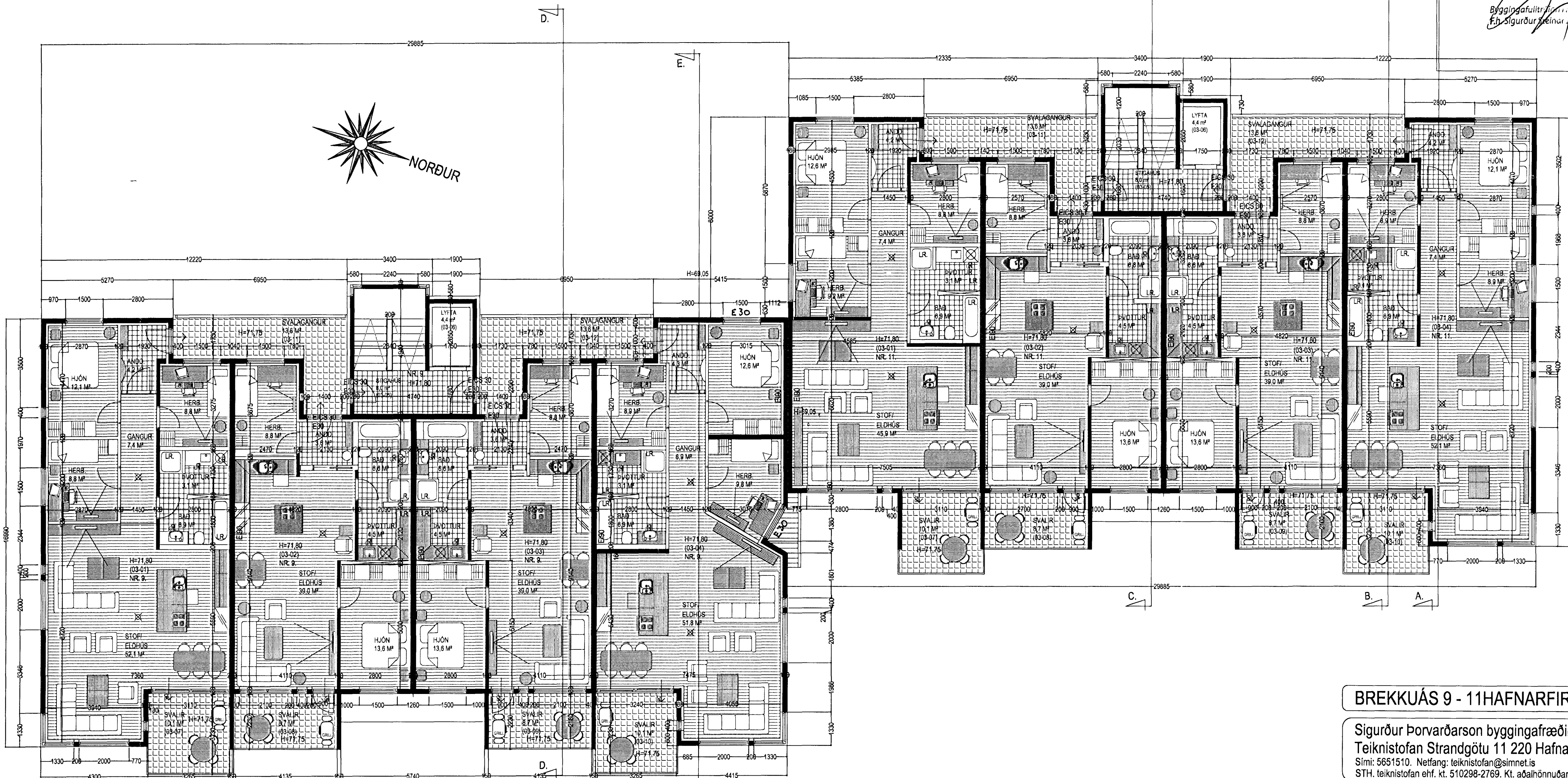
GRUNNMYND 3. HÆÐ MKV. 1:100.
