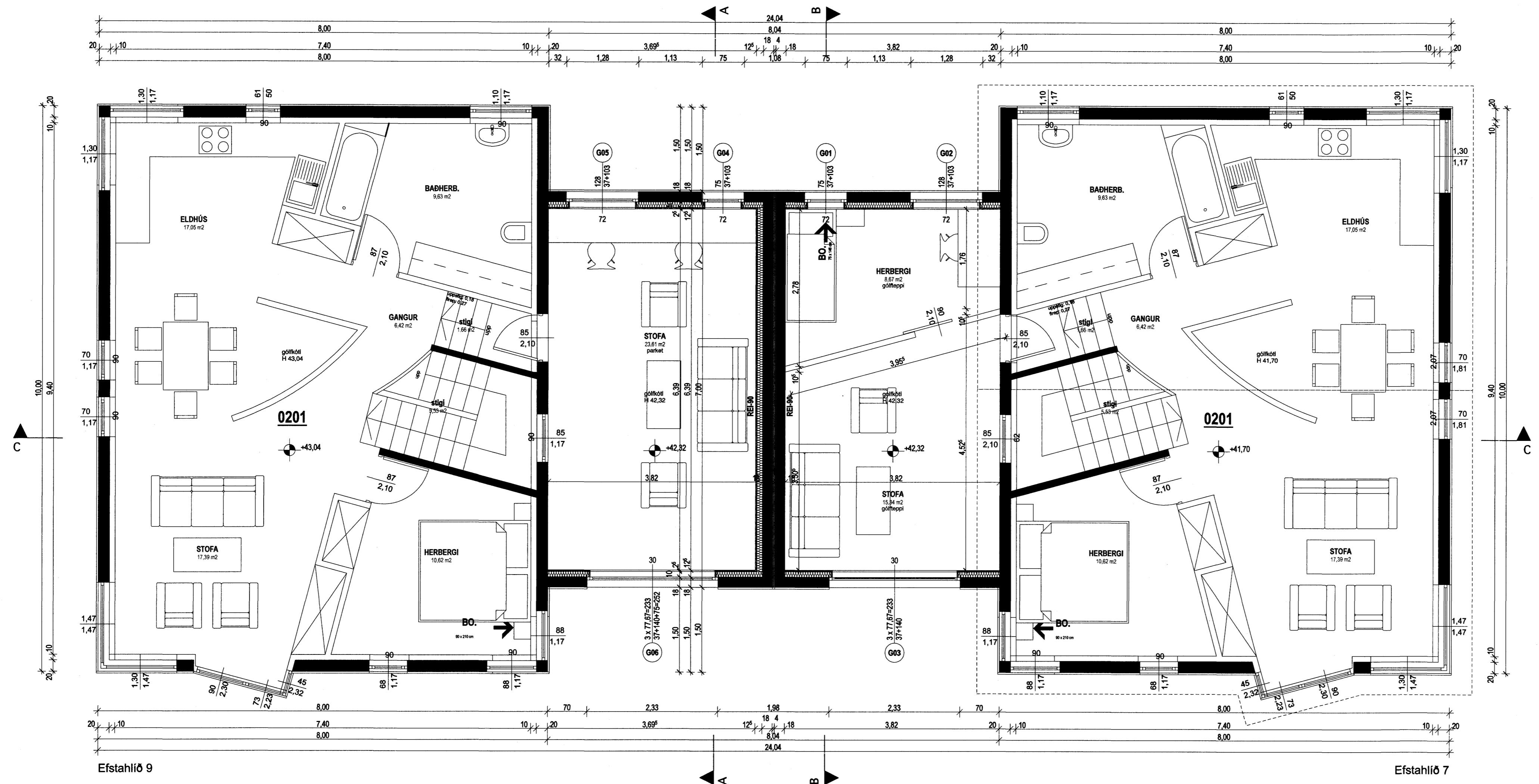
GRUNNMYND 2. HÆÐ GRUNNMYND 2. HÆÐ
