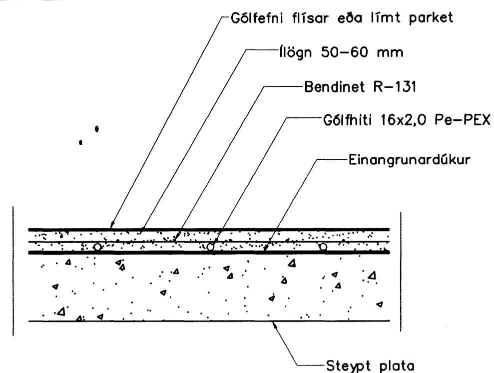
Gólfhiti snið, 1:10
