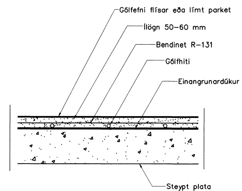
Gólfhiti snið, 1:10
