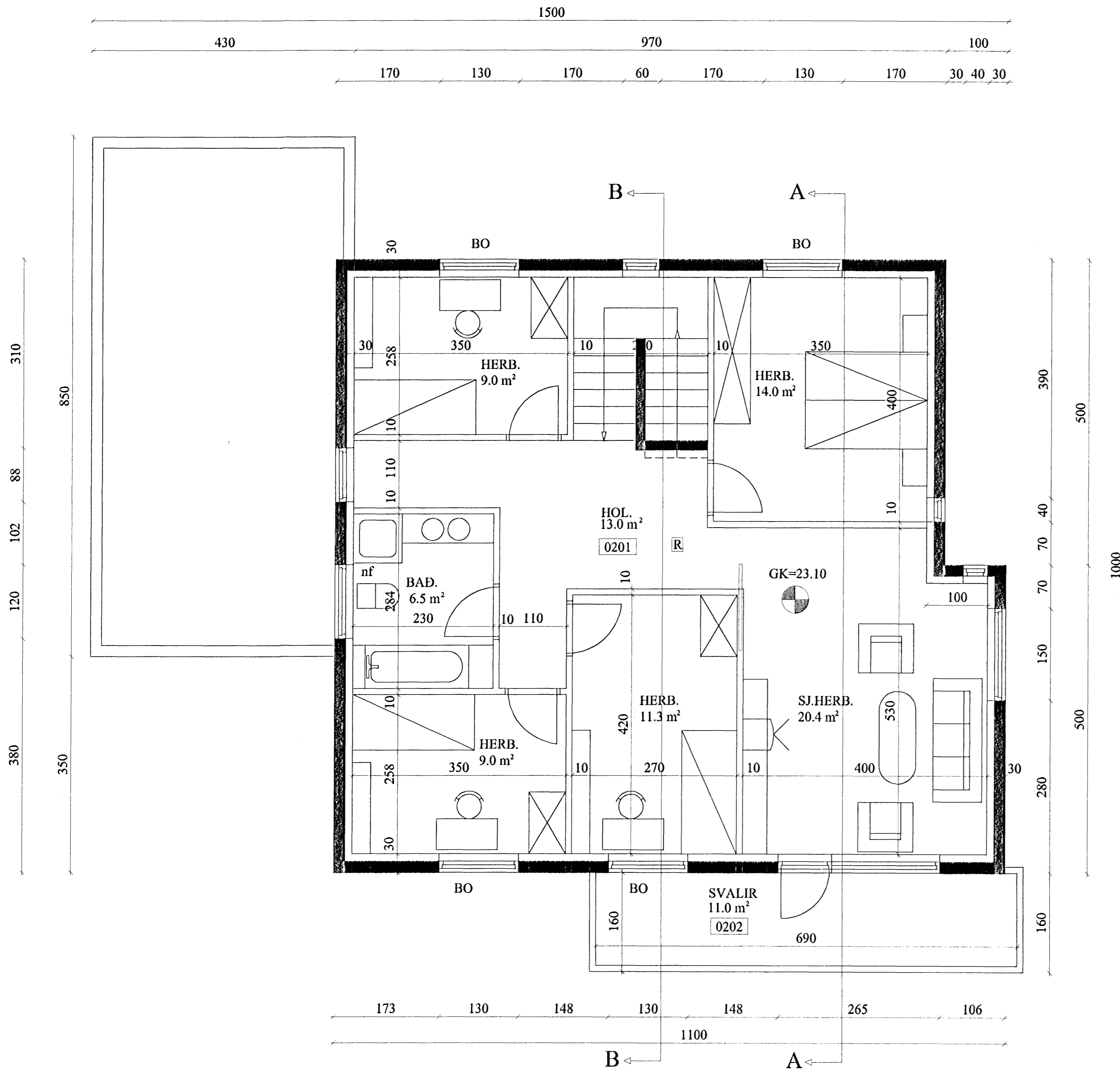
GRUNNMYND 2.HÆÐ.
