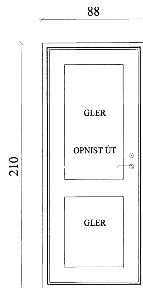
HURÐASPJALD 80 MÁL TAKIST Á STAÐNUM G 8. 1.stk. svalahurð
