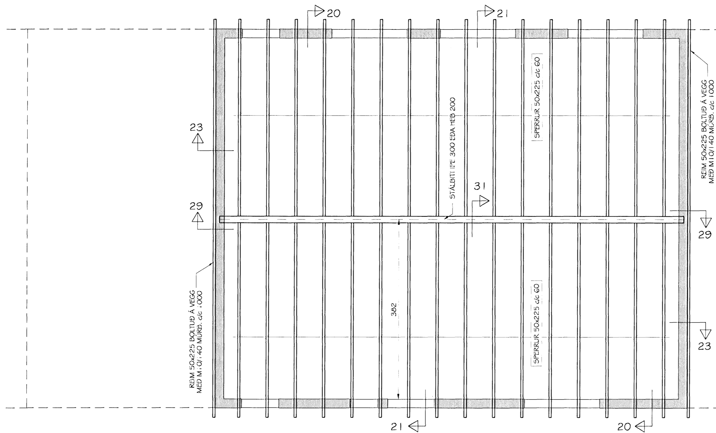
BLÓMVELLIR 29 GRUNNMYND ÞAKVIÐA MKV. 1:50
