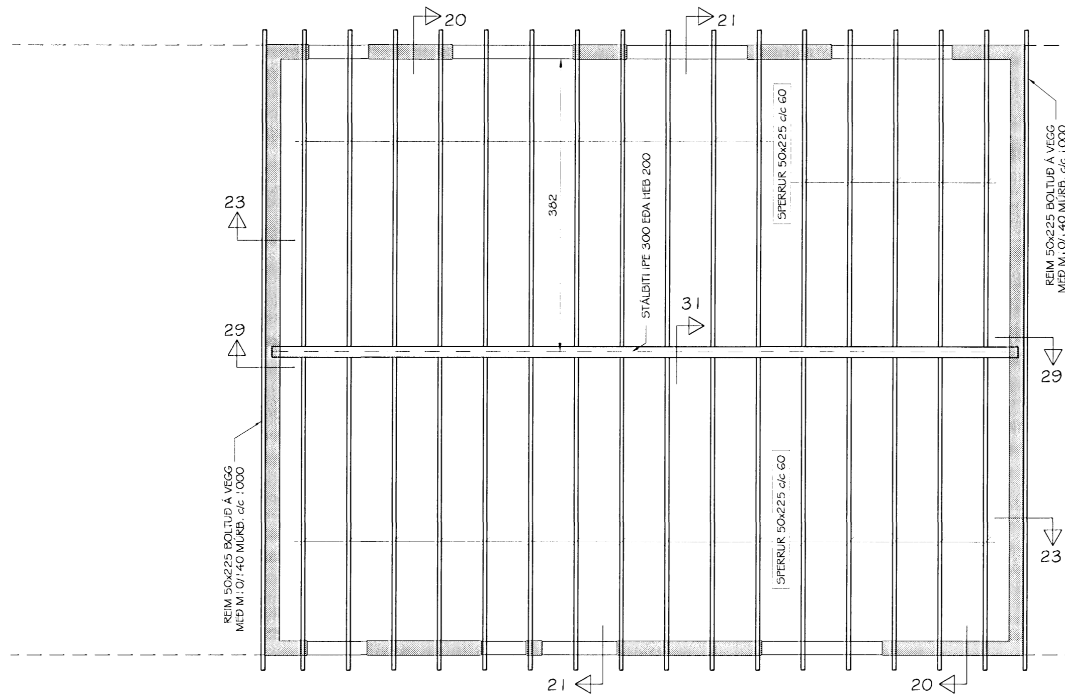
BLÓMVELLIR 31 GRUNNMYND ÞAKVIÐA MKV. 1:50
