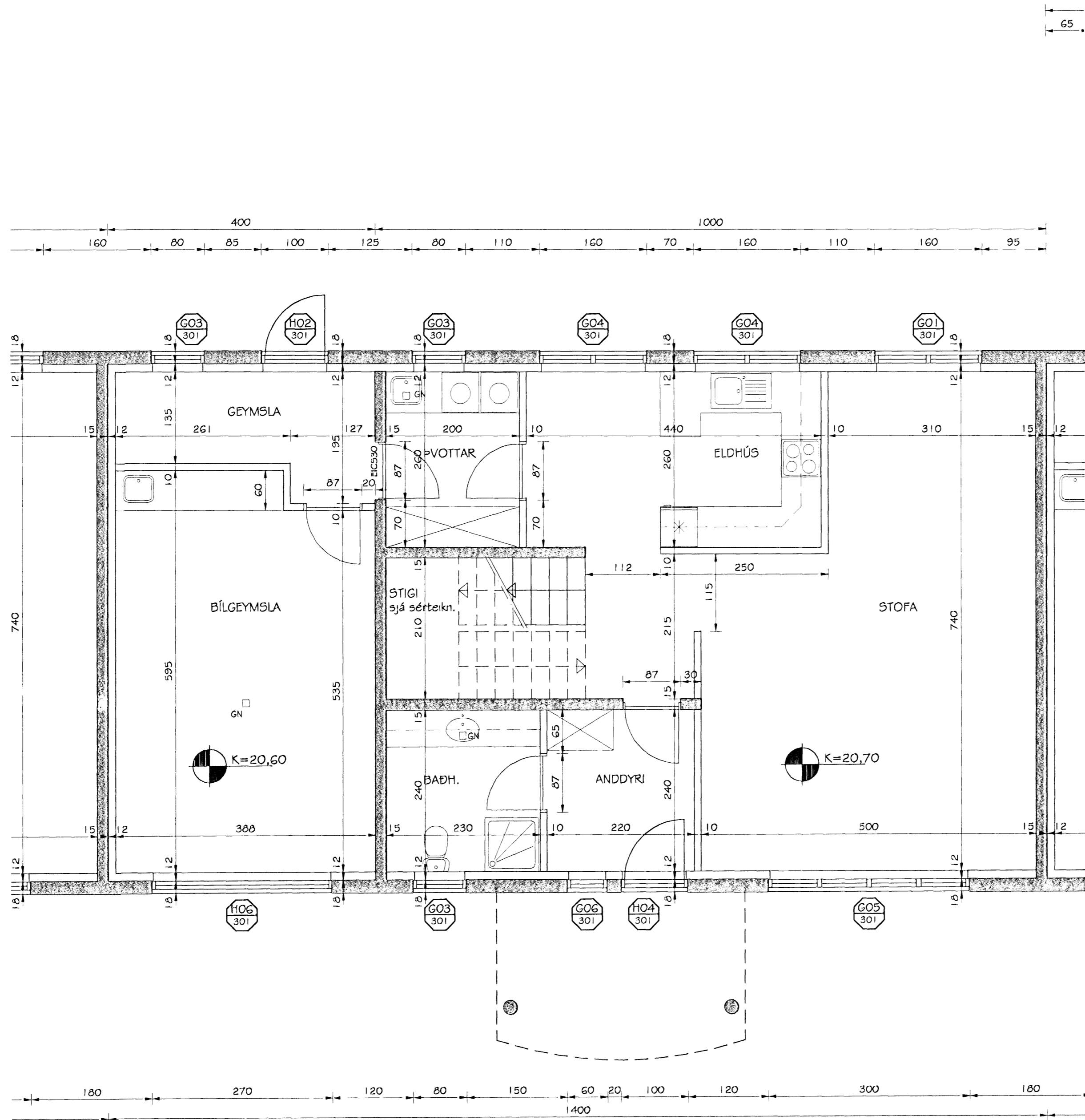
BLÓMVELLIR 33 GRUNNMYND NEDRI HÆÐAR MKV. 1:50
