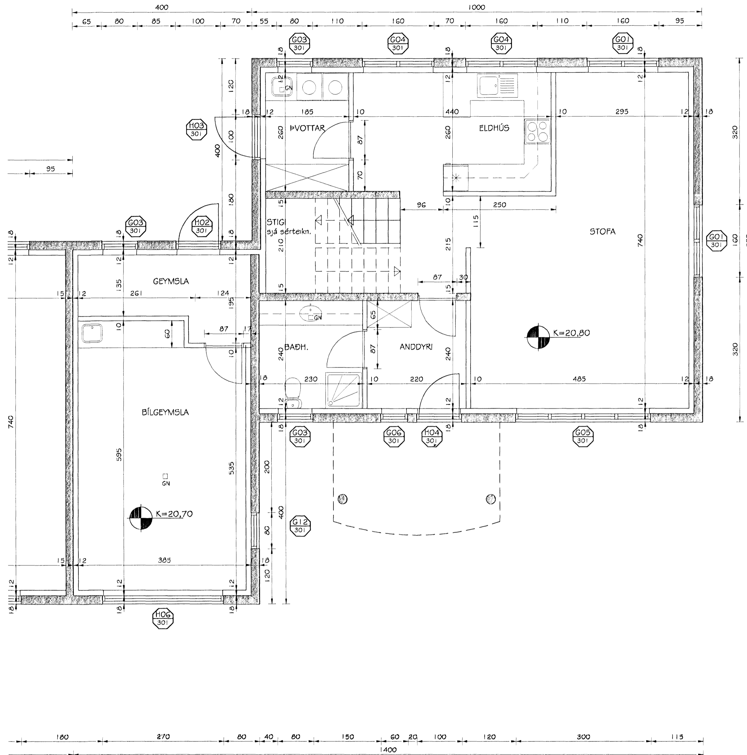
BLÓMVELLIR 35 GRUNNMYND NEDRI HÆÐAR MKV. 1:50
