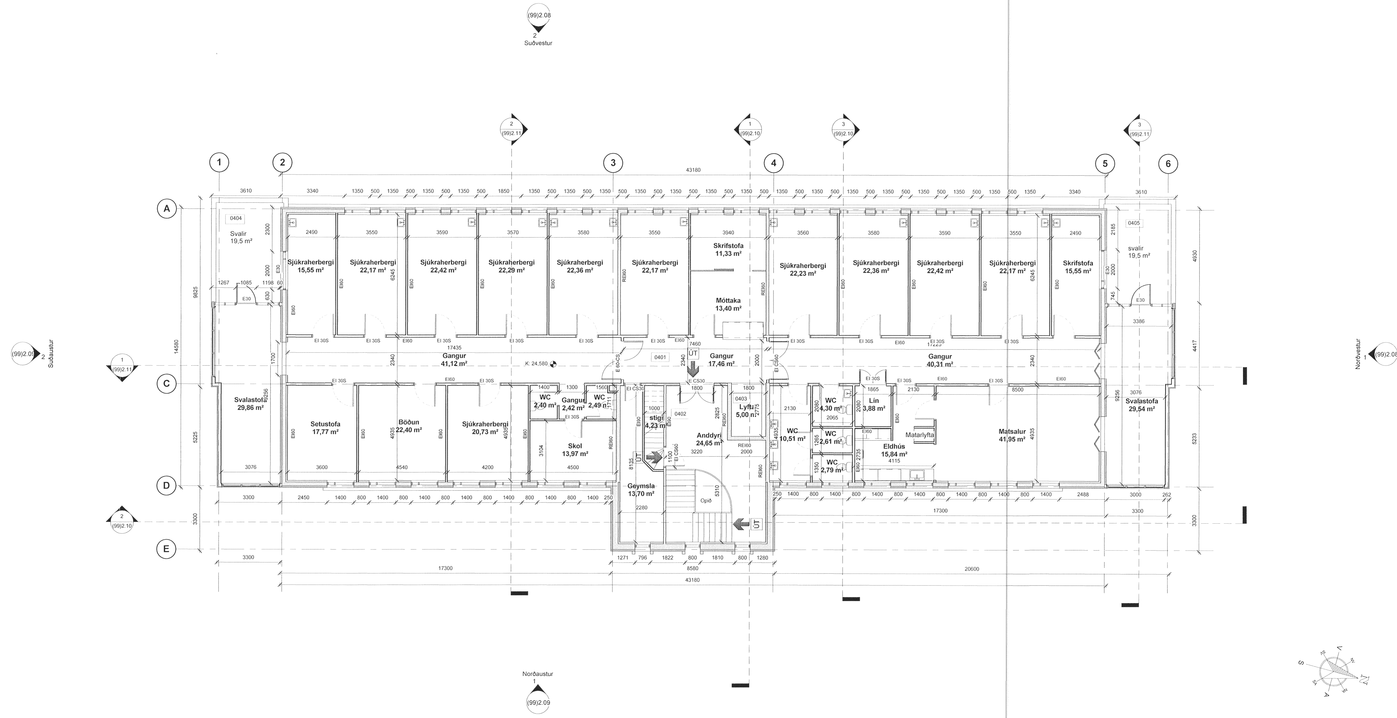
1 4.hæð 1:100
