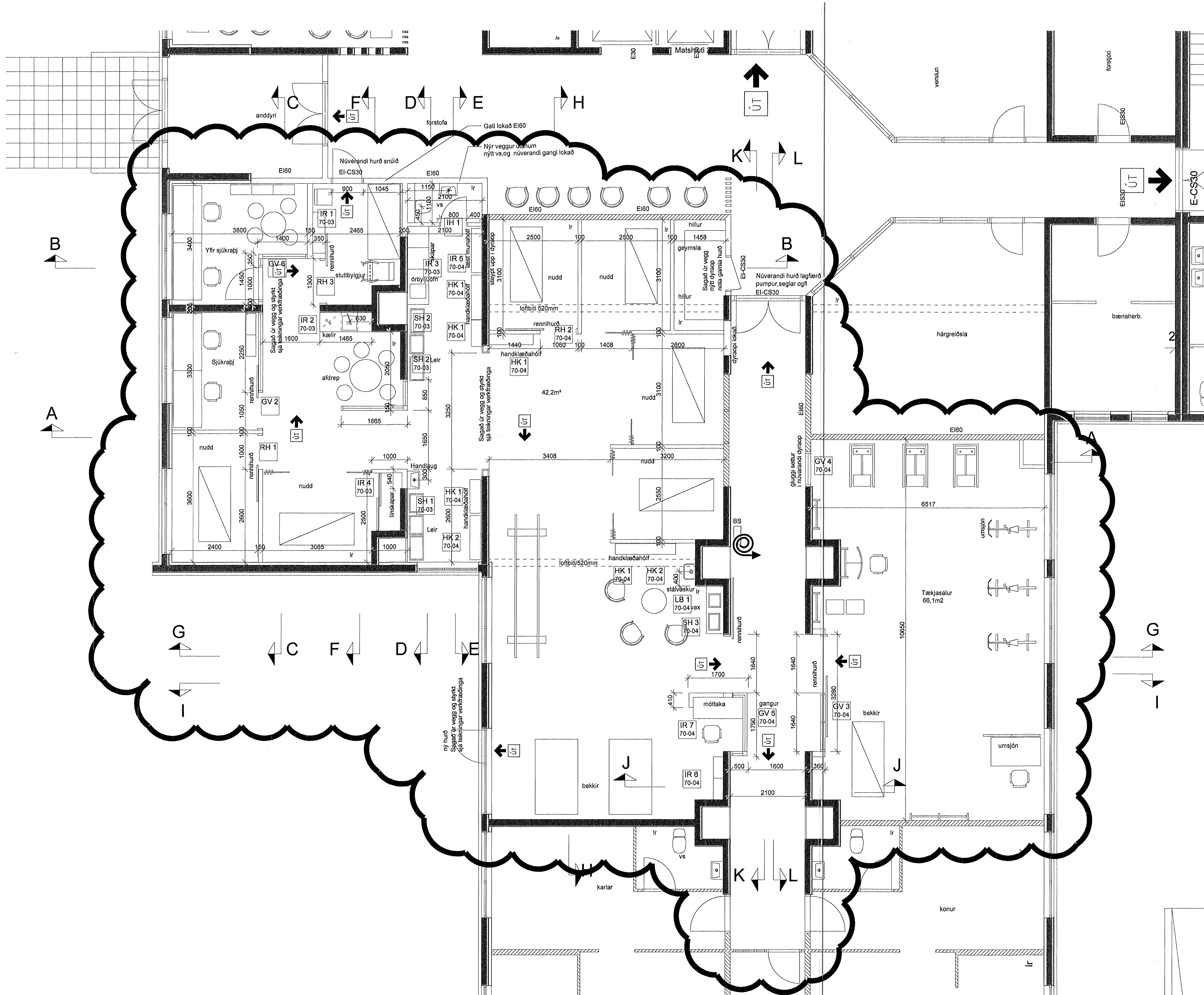
GRUNNMYND SJUKRÁLFJUN 1. HÆÐ B-ÁLMI 1:50
