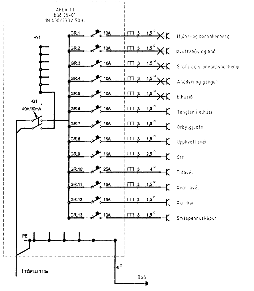
Einlínnumyndir 5.hæð
