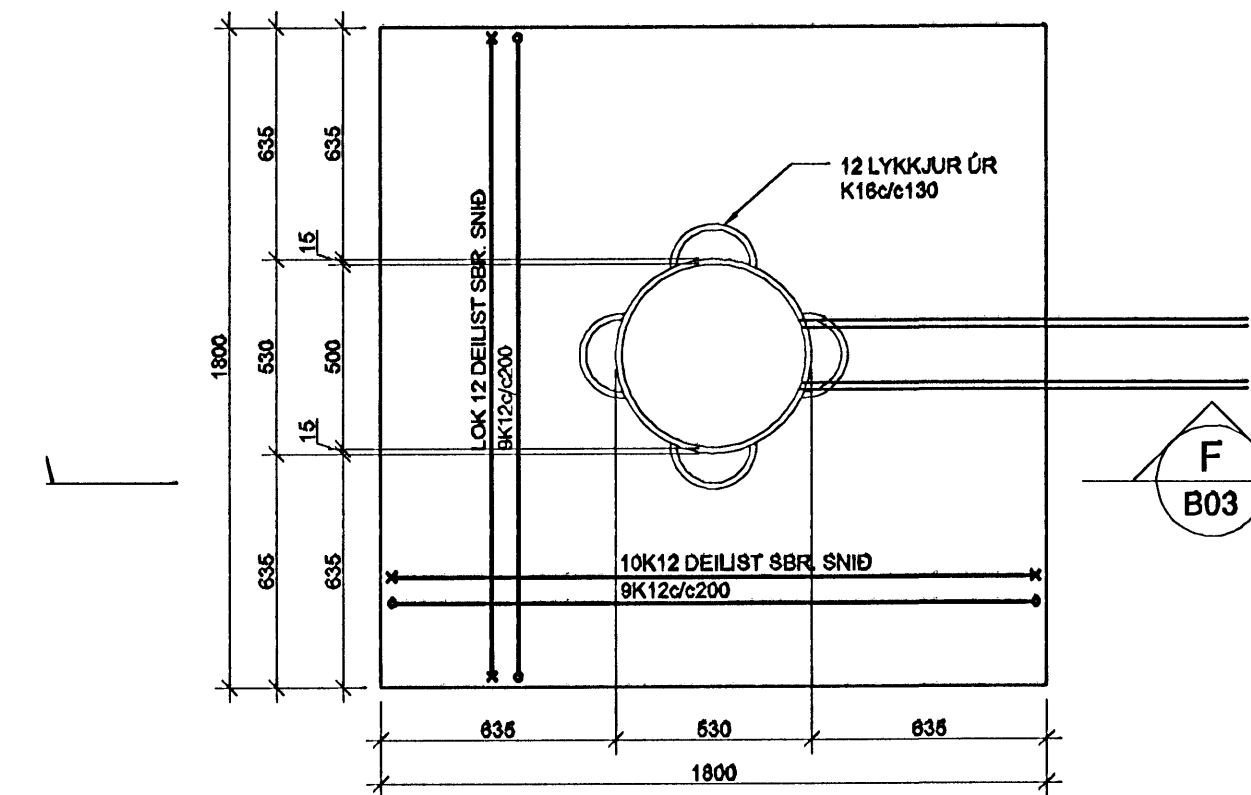
GRUNNMYND JÓLATRÉSFÓTAR 1:20
