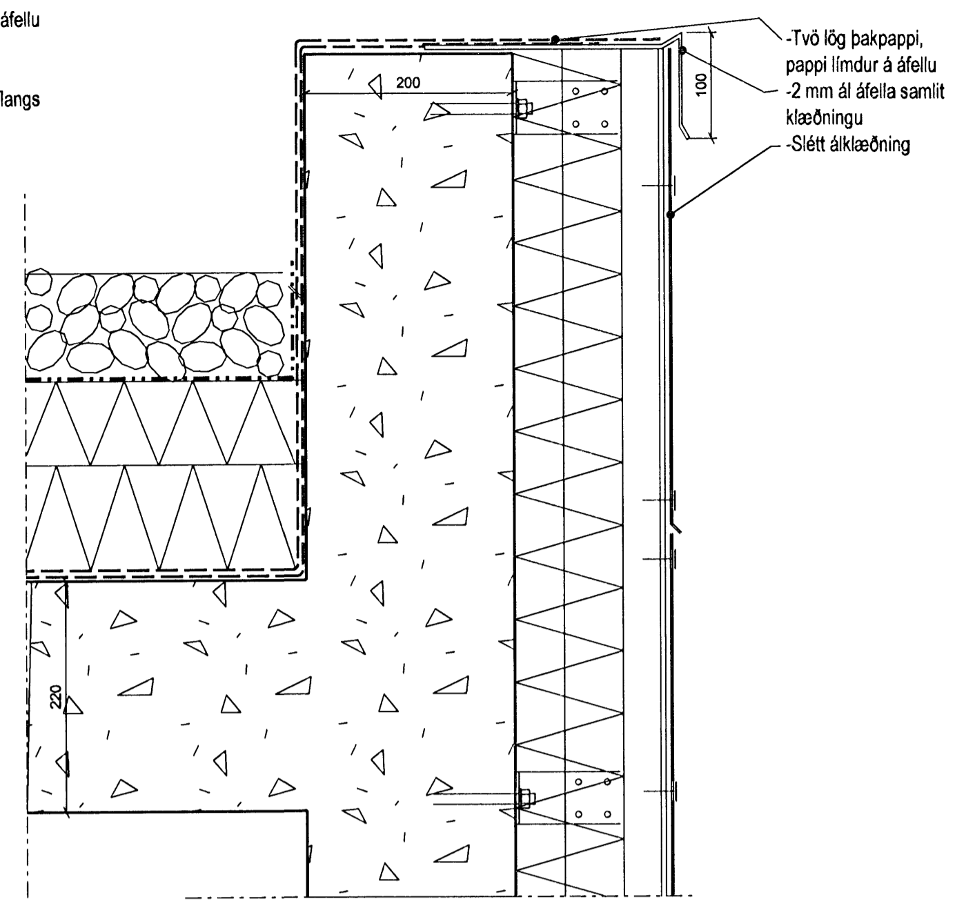
3 DEILI 1:5 Þakfrágangur, almenn, slétt klæðning
