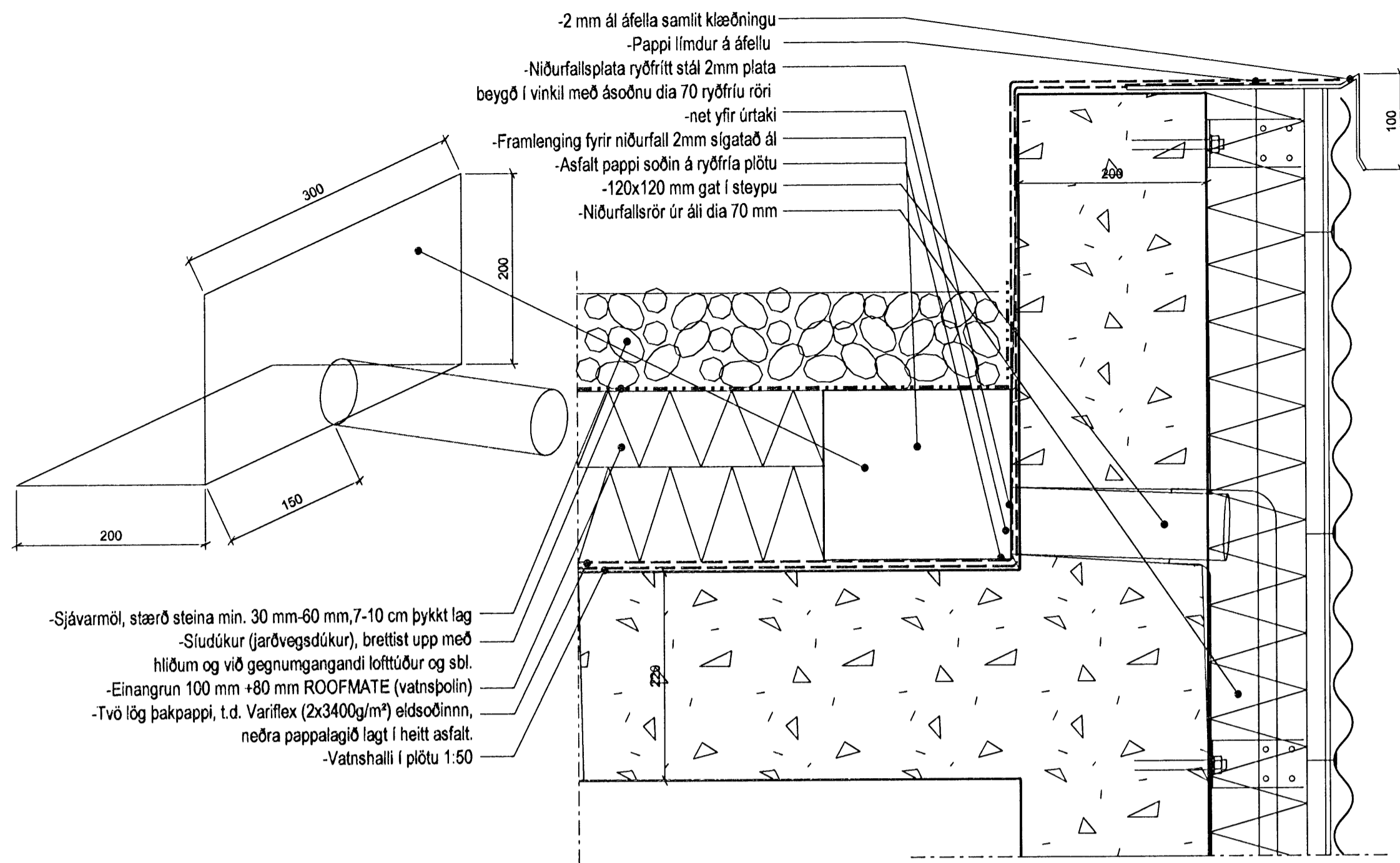
1 DEILI 1:5 Þakfrágangur niðurfall
