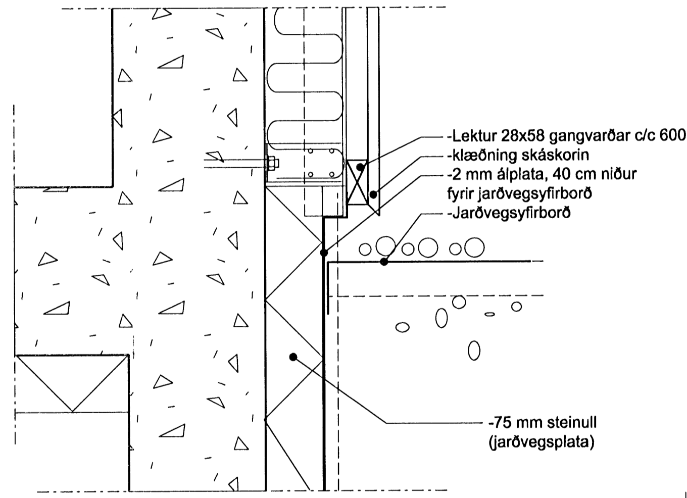
6 DEILI 1:5 Frágangur við sökkul, lóðrétt viðarklæðning
