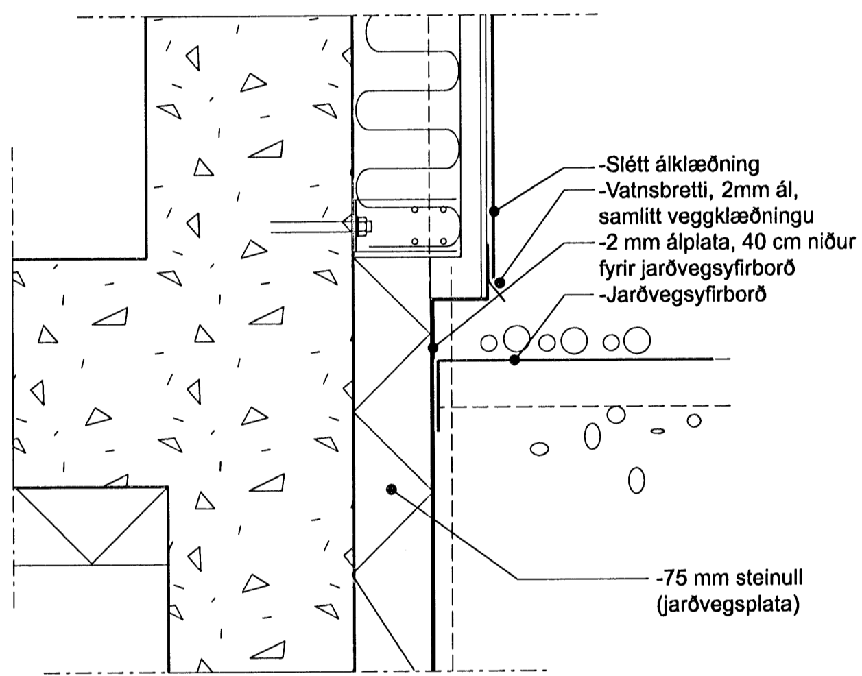
5 DEILI 1:5 Frágangur við sökkul, slétt álklæðning
