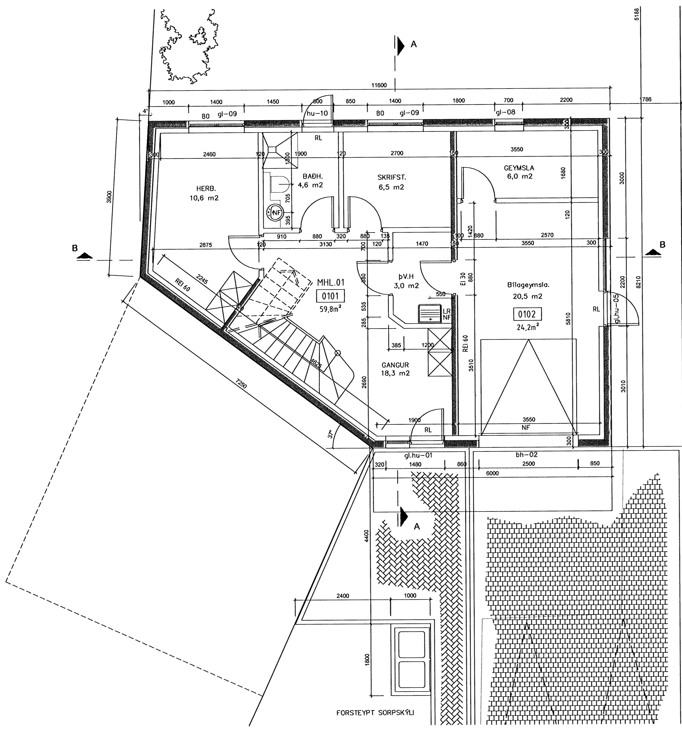
GRUNNMYND 1. HÆÐAR 1:50
