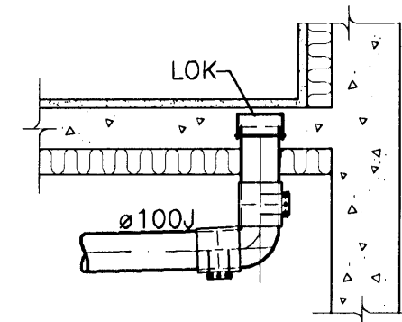
FRÁGANGUR GÓLFSTÚTS TIL FRAMTÍDARTENGINGAR
