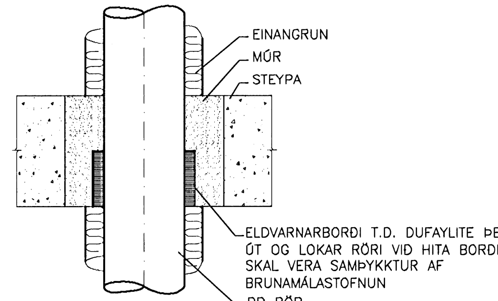
BRUNAPÉTTING Á PP LEIDSLU GEGNUM STEYPT GÓLF
