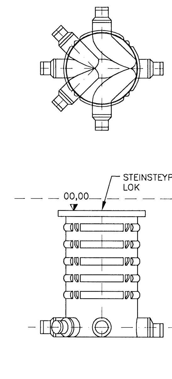
PLASTBRUNNUR ø600
