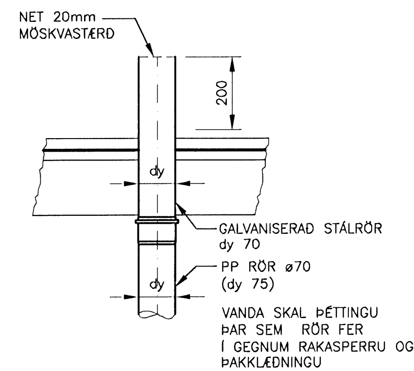
ÚTLOFTUN UPP ÚR ÞAKI
