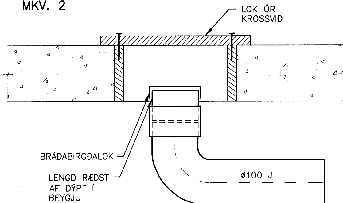
FRÁGANGUR GÓLFSTÚTA
