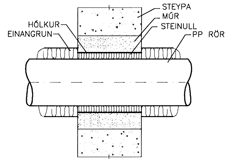
ÞÉTTING Á PP LEIDSLU GEGNUM STEYPTAN VEGG
