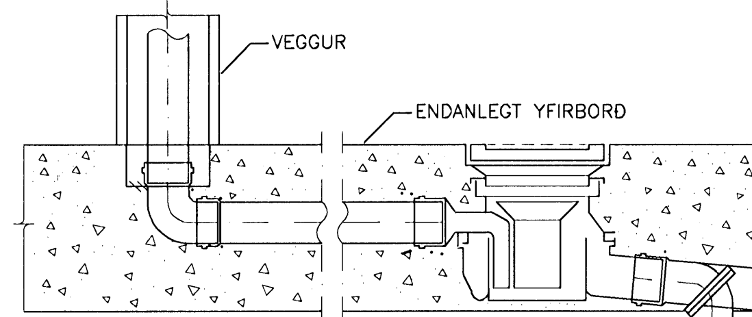
GÓLFNIDURFALL MED GEGNUMRENSSLI Í GRUNNPLÖTU
