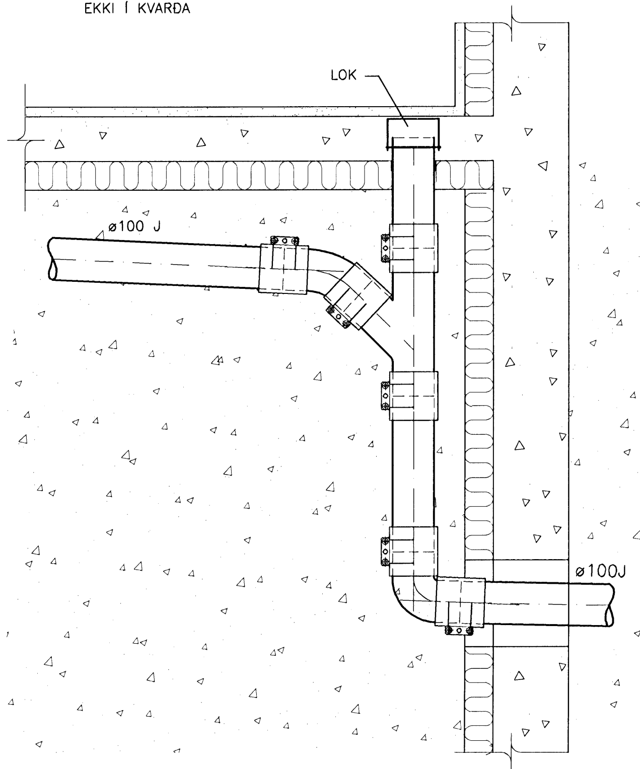
FALLPIPA Í GRUNNI
