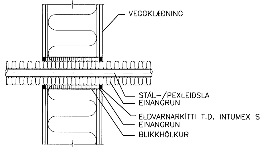
BRUNAPÉTTING Á STÁL-/PEXLEIDSLU GEGNUM LÉTTAN VEGG
