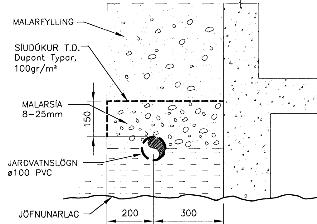
FRÁGANGUR JÄRVATNSLAGNAR ÚR PVC
