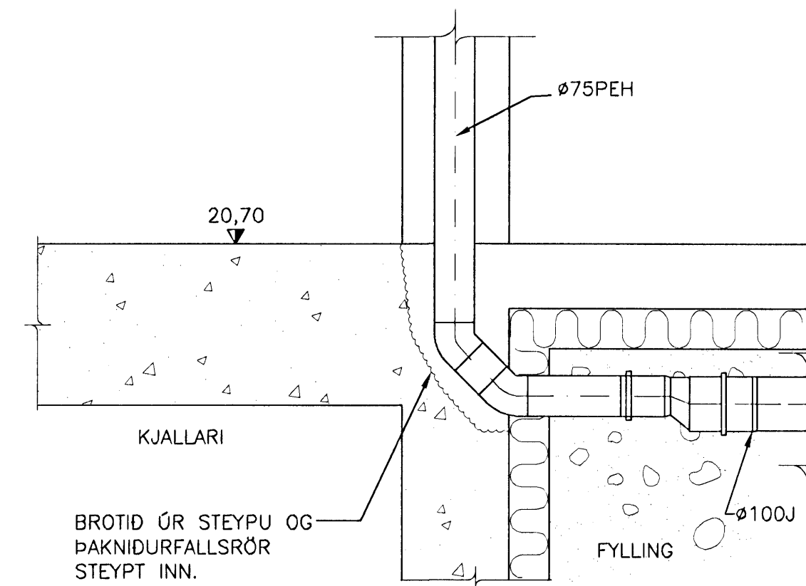
INNSTEYPT ÞAKNIDURFALL
