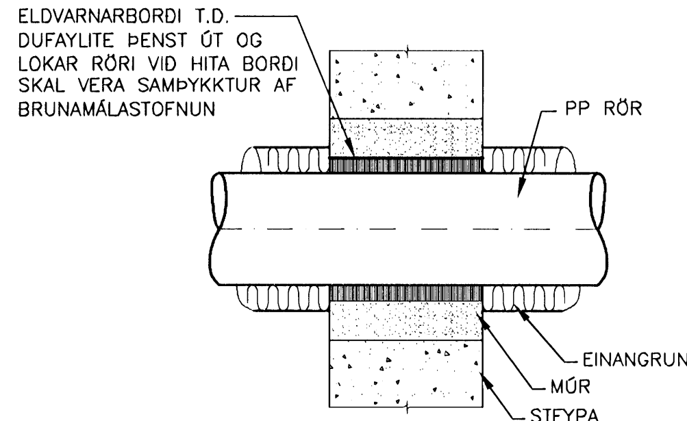
BRUNAPÉTTING Á PP LEIDSLU GEGNUM STEYPTAN VEGG
