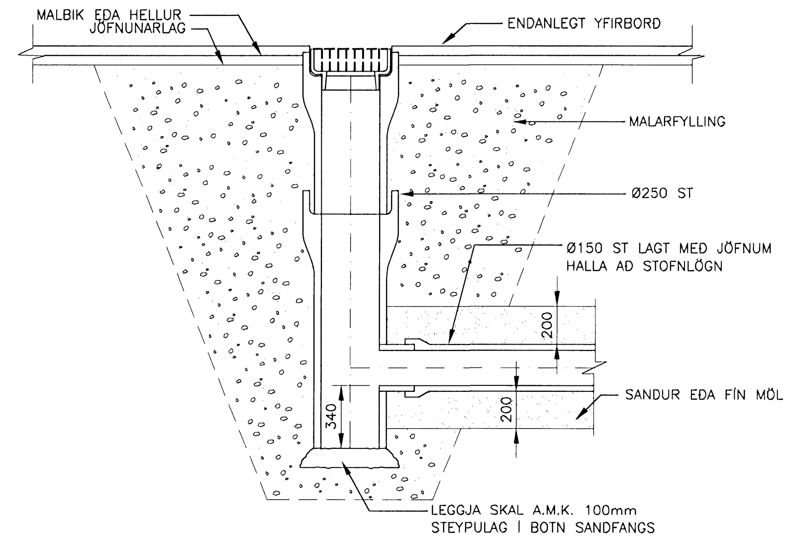
FRÁGANGUR Á GÖTUNIDURFALLI
