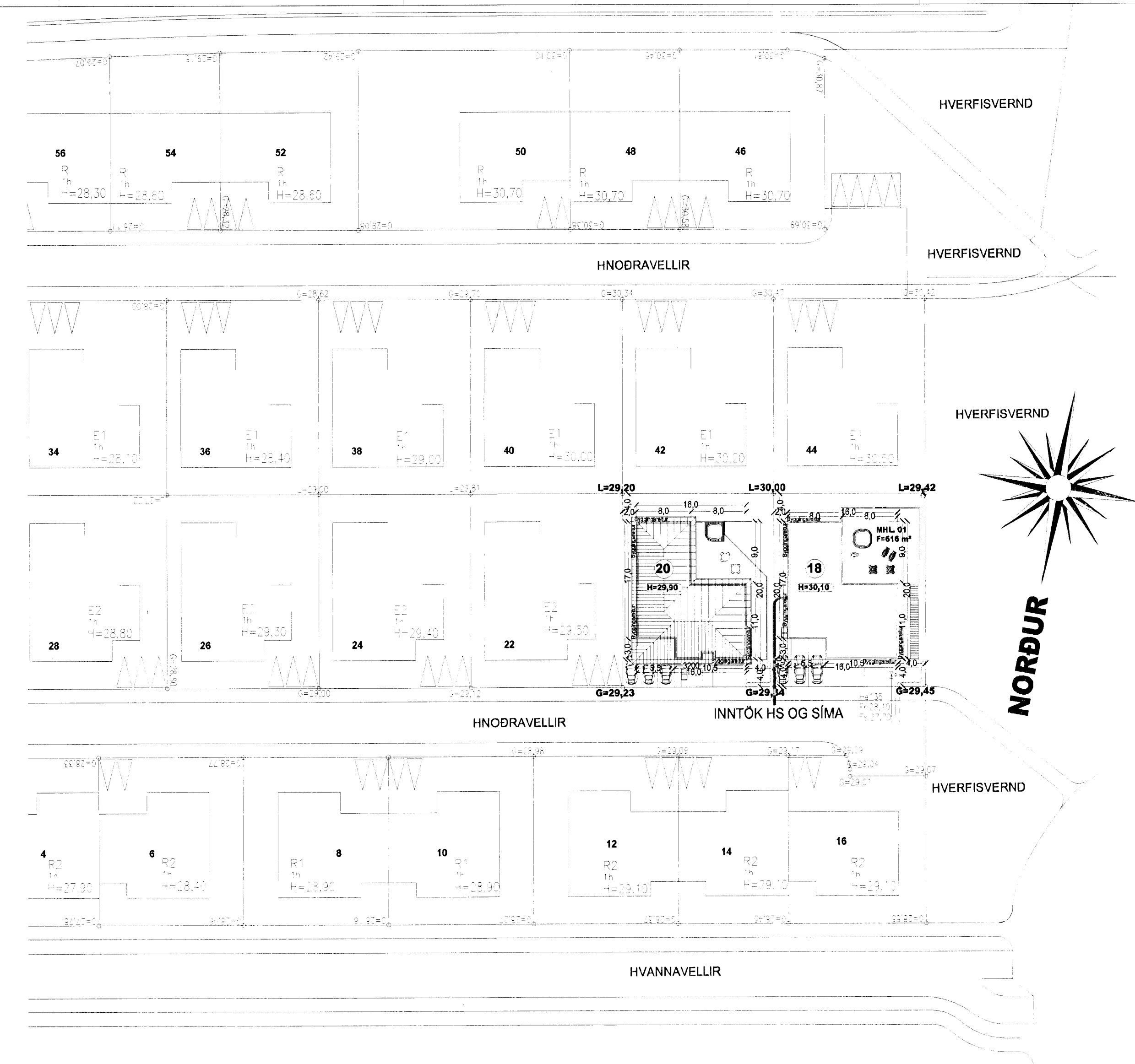
AFSTÖÐUMYND MKV. 1:500
