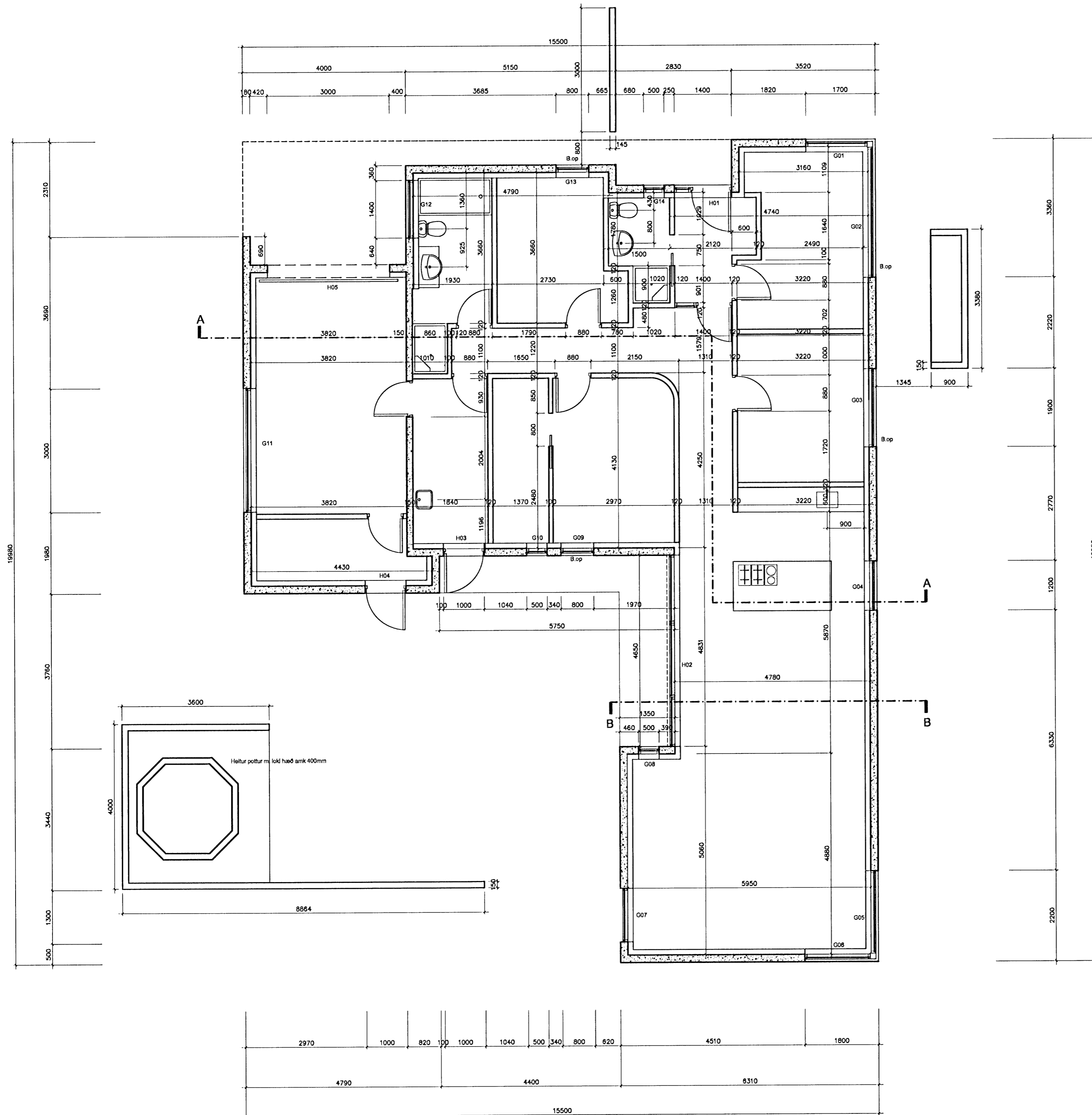
Grunnmynd 1:50
