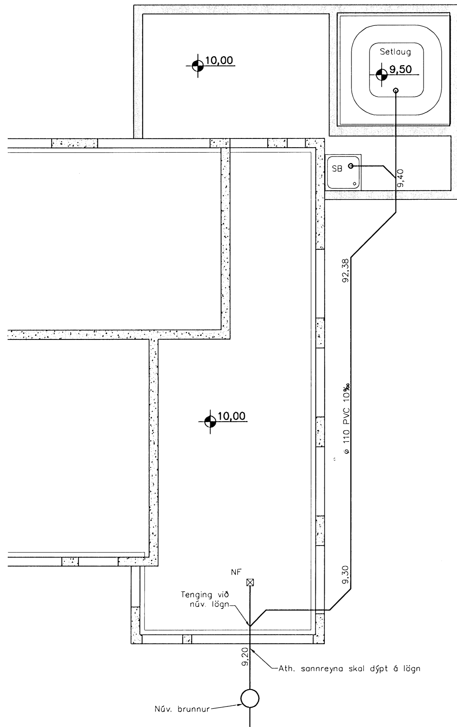
Grunnlagnir 1:50
