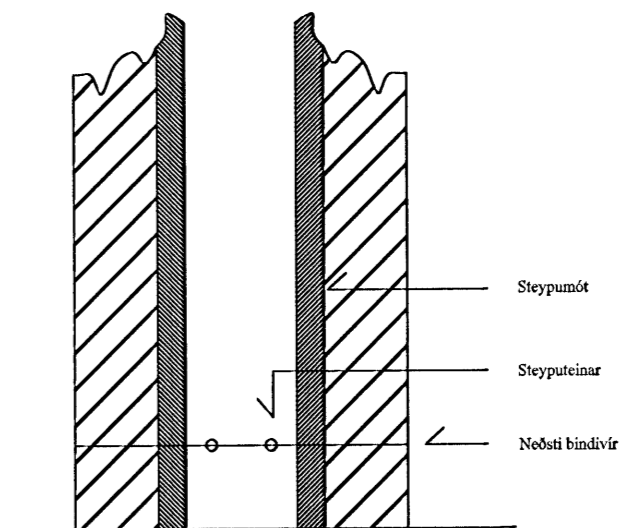
Snið í sökkulvegg
