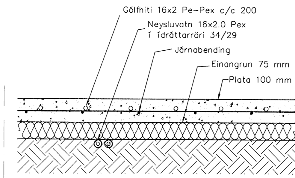
Hita- og vatnslagnir. Snið í botnplötu, 1:10
