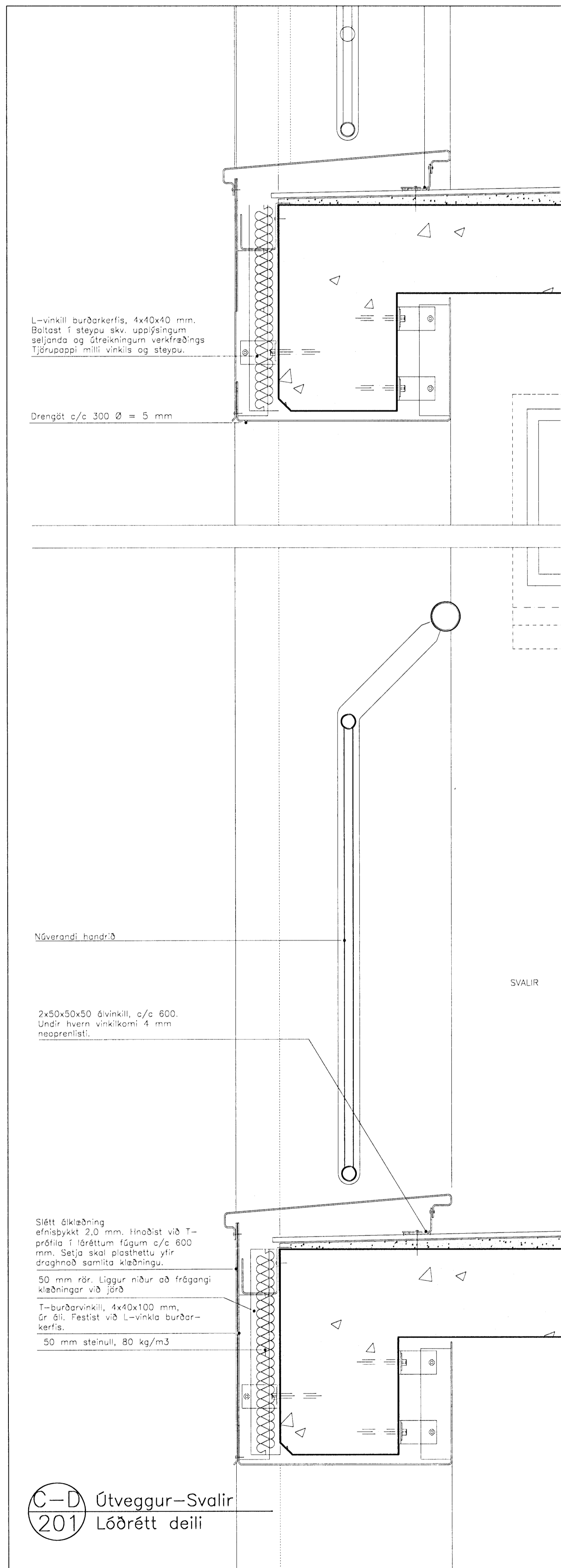
C-D Útveggur-Svalir-Lokun 201 Lóðrétt deili
