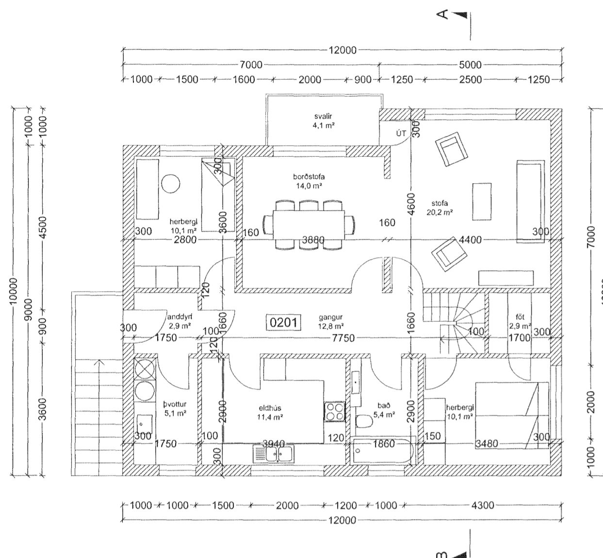
grunnmynd 2. hæð
