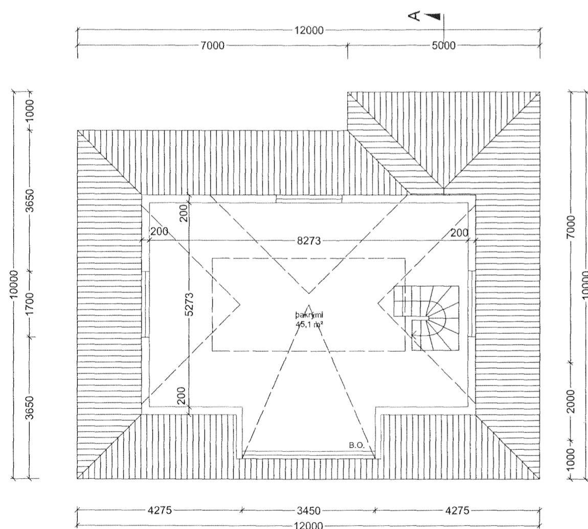
grunnmynd þakhæð
