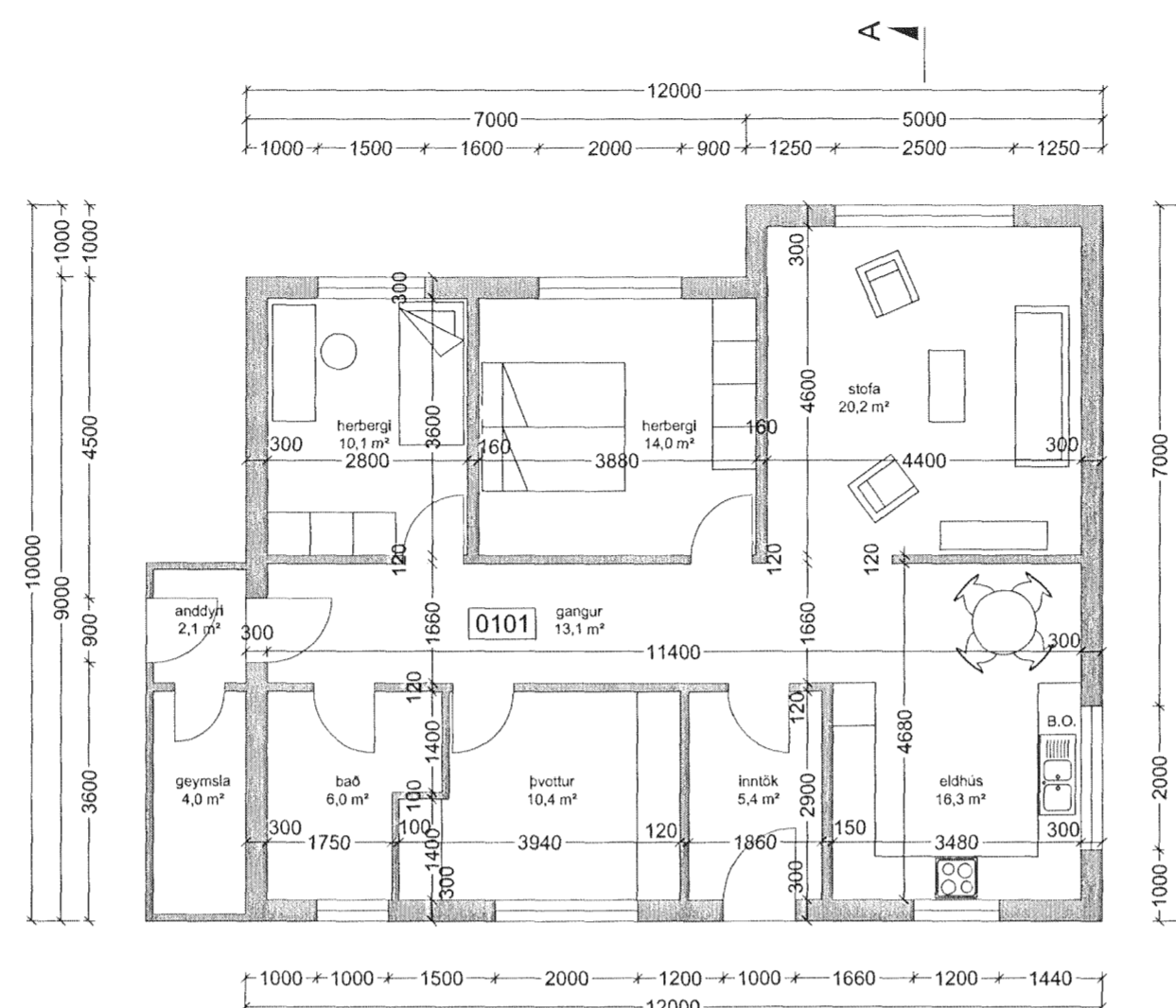
grunnmynd 1. hæð
