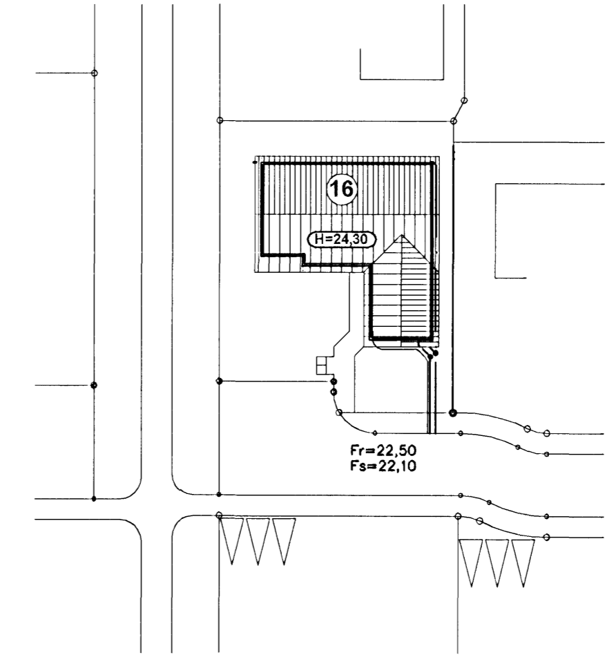
Afstöðumynd 1:500
